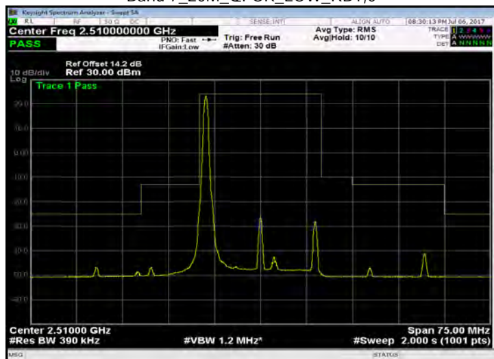
Band 7_20M_QPSK_LOW_RB1,99
