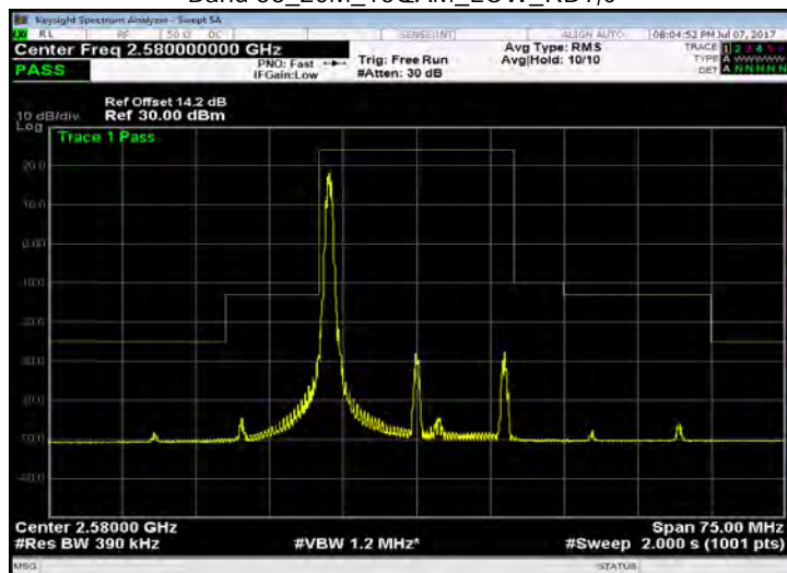
Band 38_20M_16QAM_LOW_RB1,99
