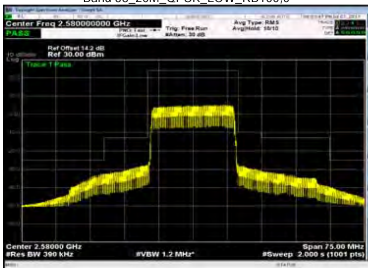
Band 38_20M_QPSK_LOW_RB100,0
