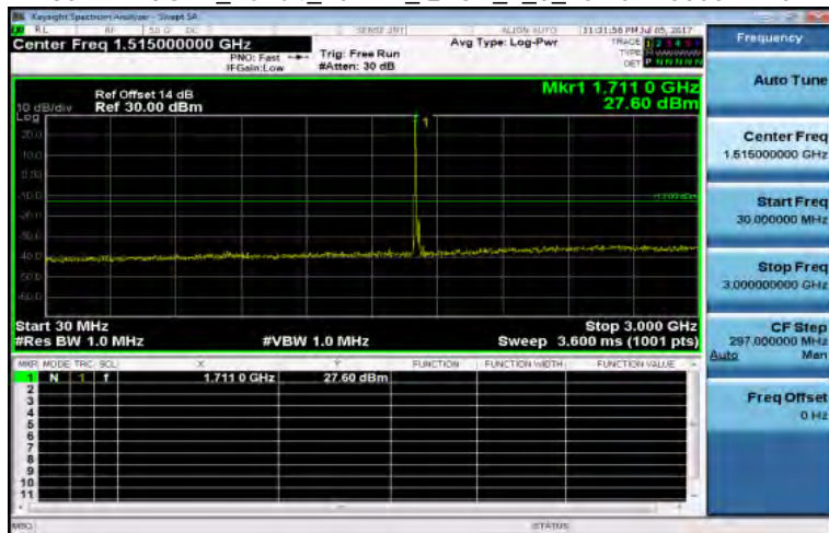
30MHz~3GHz_Band4_20MHz_QPSK_1_0_LowCH20050-1720
