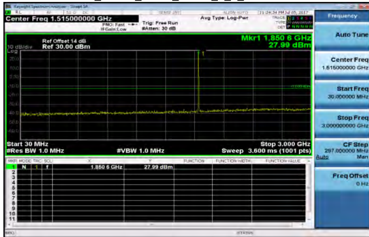
30MHz~3GHz_Band2_3MHz_QPSK_1_0_LowCH18615-1851.5
