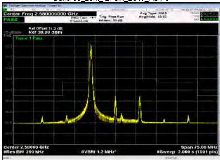
Band 38_20M_QPSK_LOW_RB1,99
