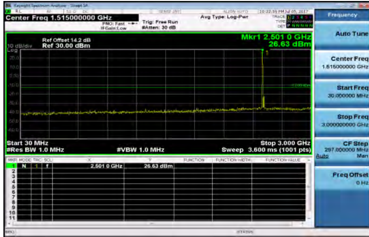
30MHz~3GHz_Band7_20MHz_QPSK_1_0_LowCH20850-2510
