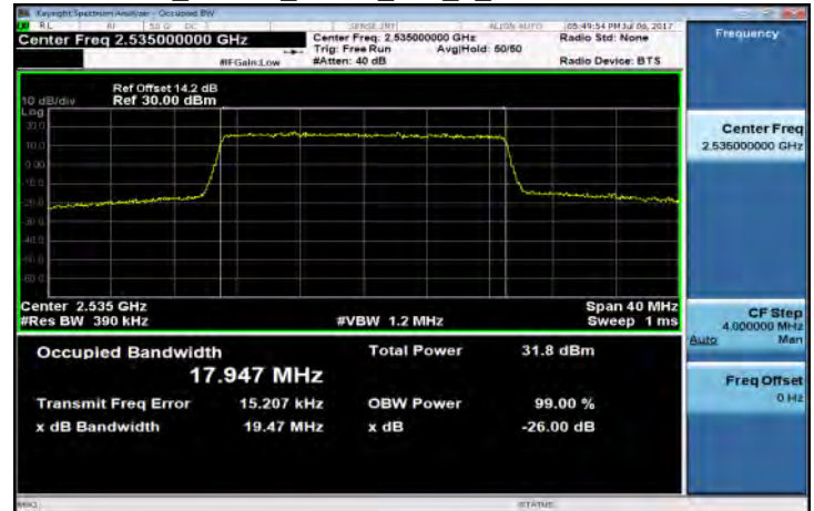
Band7_20MHz_QPSK_100_0_MidCH21100-2535
