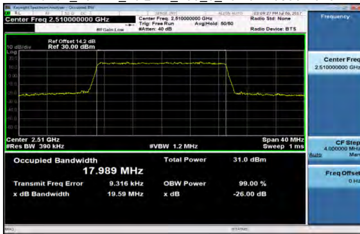
Band7_20MHz_16QAM_100_0_LowCH20850-2510
