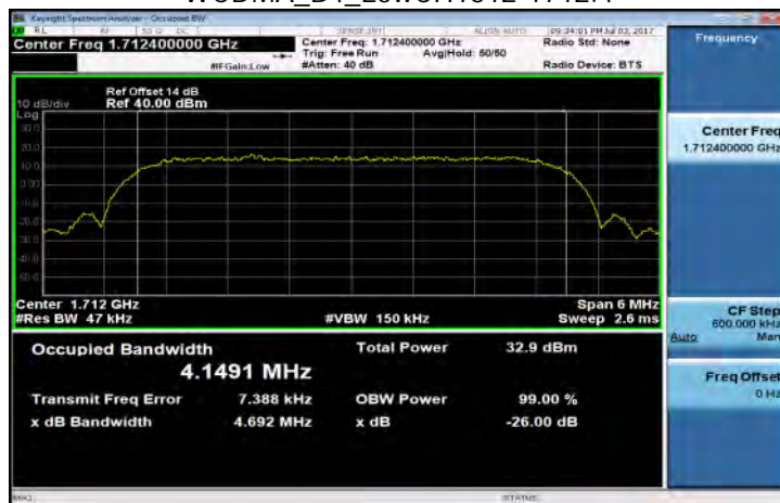
WCDMA_B4_LowCH1312-1712.4
