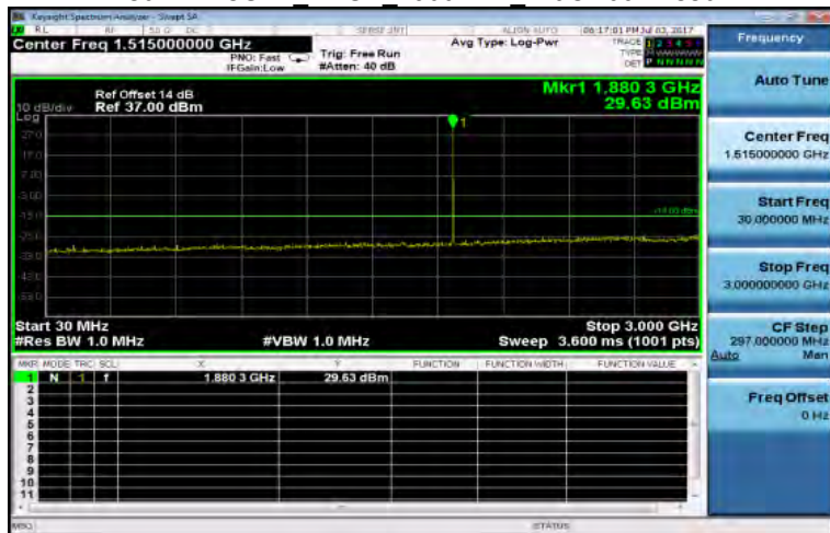
30MHz~3GHz EDGE 1900MHz MidCH661-1880
