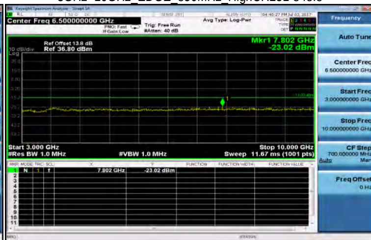
3GHz~10GHz EDGE 850MHz HighCH251-848.8
