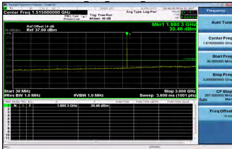
30MHz~3GHz GSM 1900MHz MidCH661-1880
