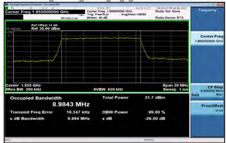
Band2_10MHz_QPSK_50_0_LowCH18650-1855
