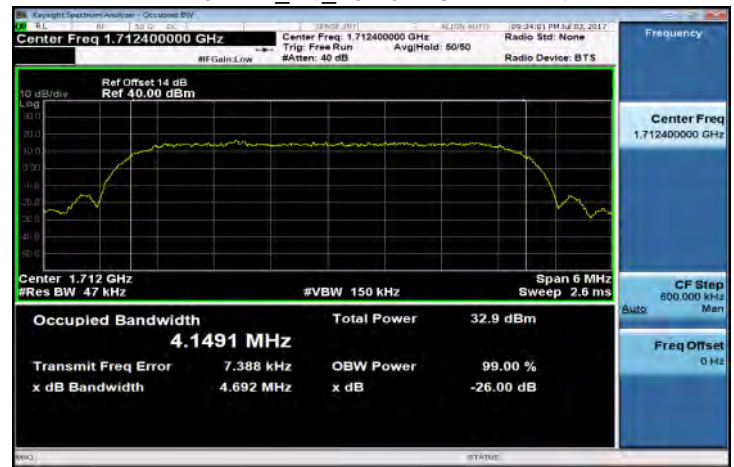
WCDMA_B4_LowCH1312-1712.4
