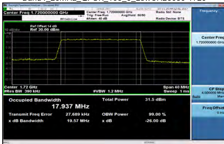
Band4_20MHz_QPSK_100_0_LowCH20050-1720
