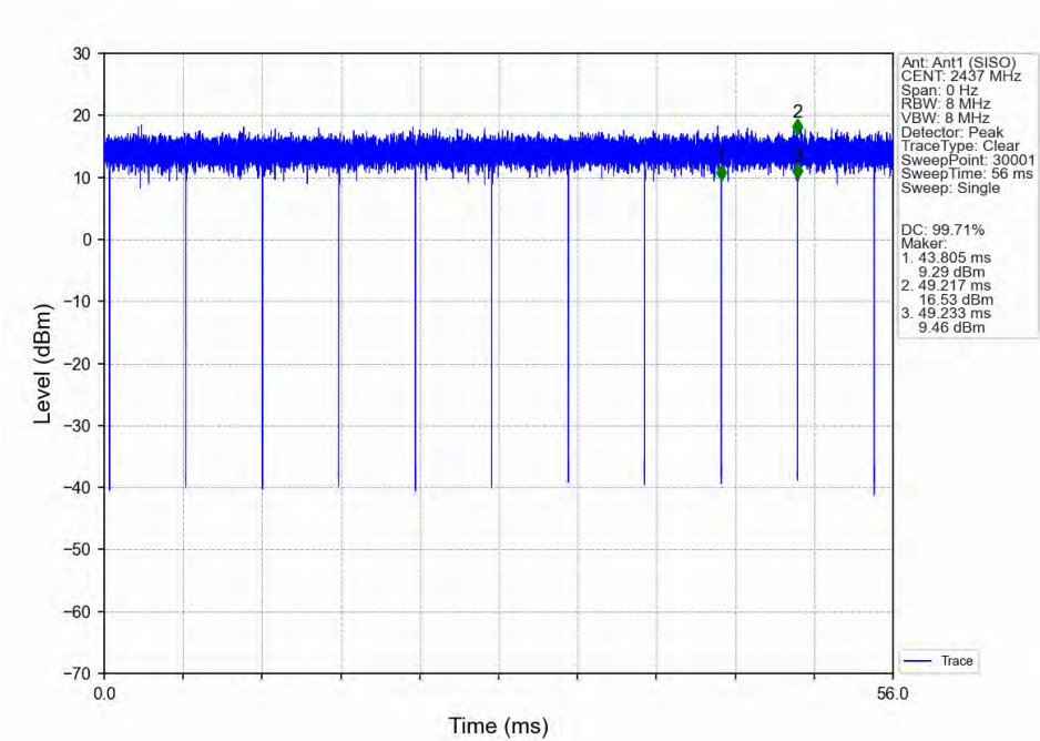
802.11n(HT40)_MCH_2437MHz_Ant1 (SISO)_NTNV
