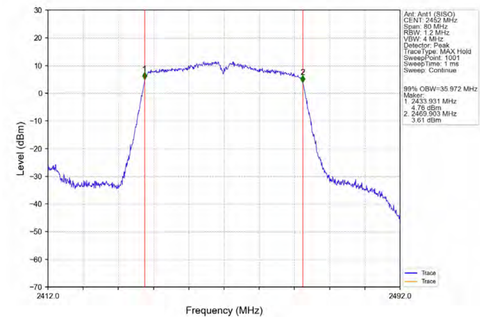
802.11n(HT40)_HCH_2452MHz_Ant1 (SISO)_NTNV
