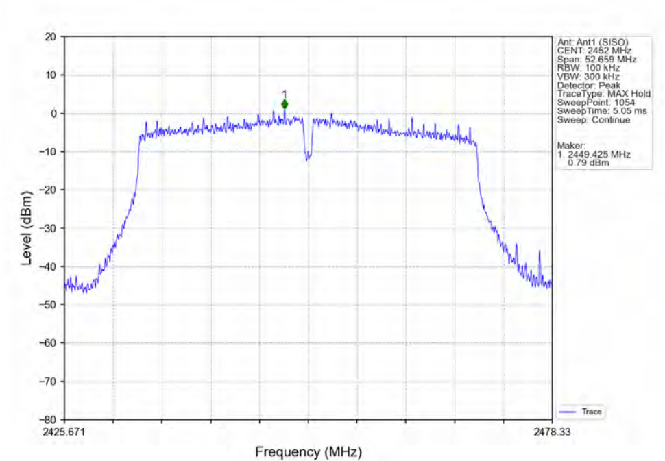
802.11n(HT40)_HCH_2452MHz_Ant1 (SISO)_NTNV
