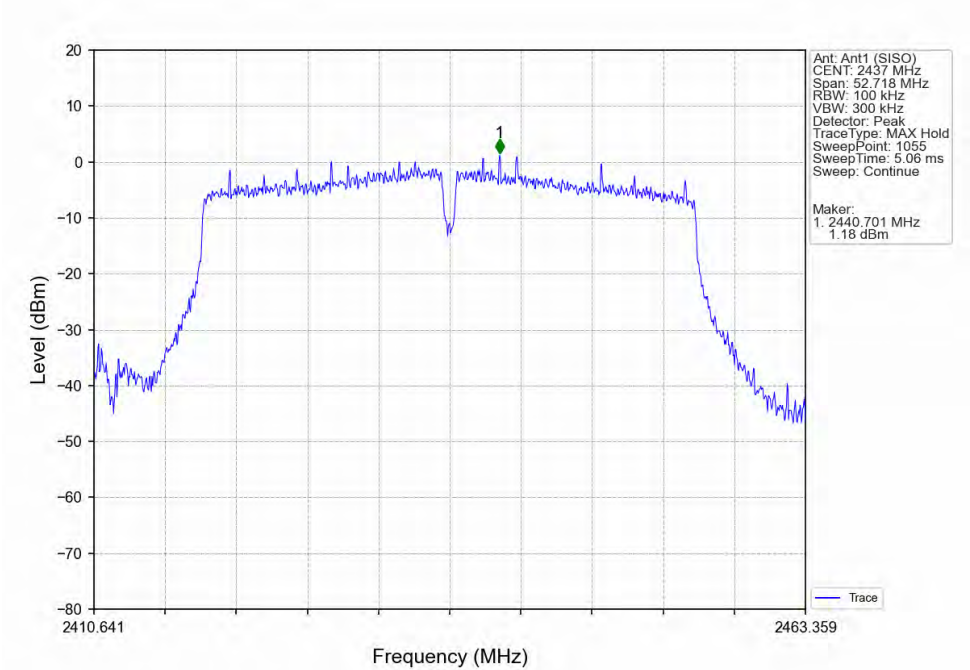
802.11n(HT40)_MCH_2437MHz_Ant1 (SISO)_NTNV
