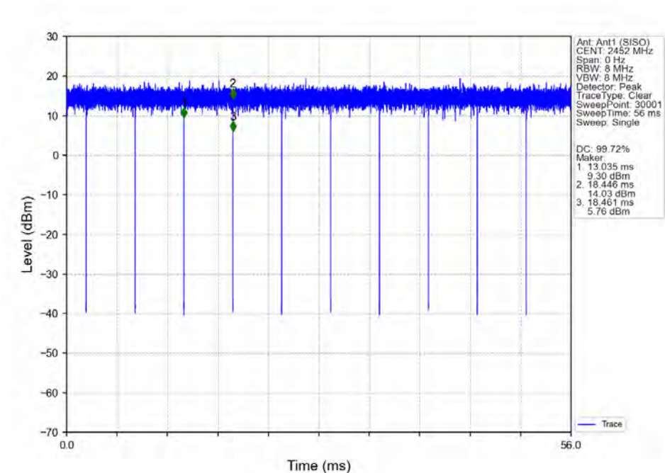
802.11n(HT40)_HCH_2452MHz_Ant1 (SISO)_NTNV
