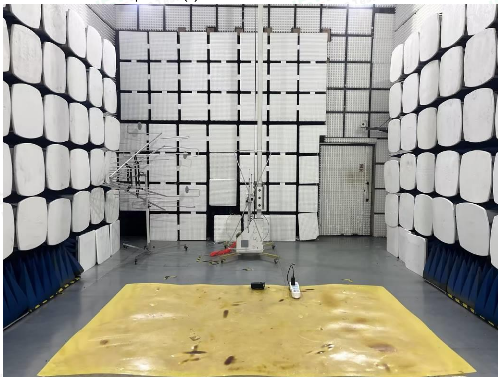
Fig. 1 (30MHz~1GHz)
