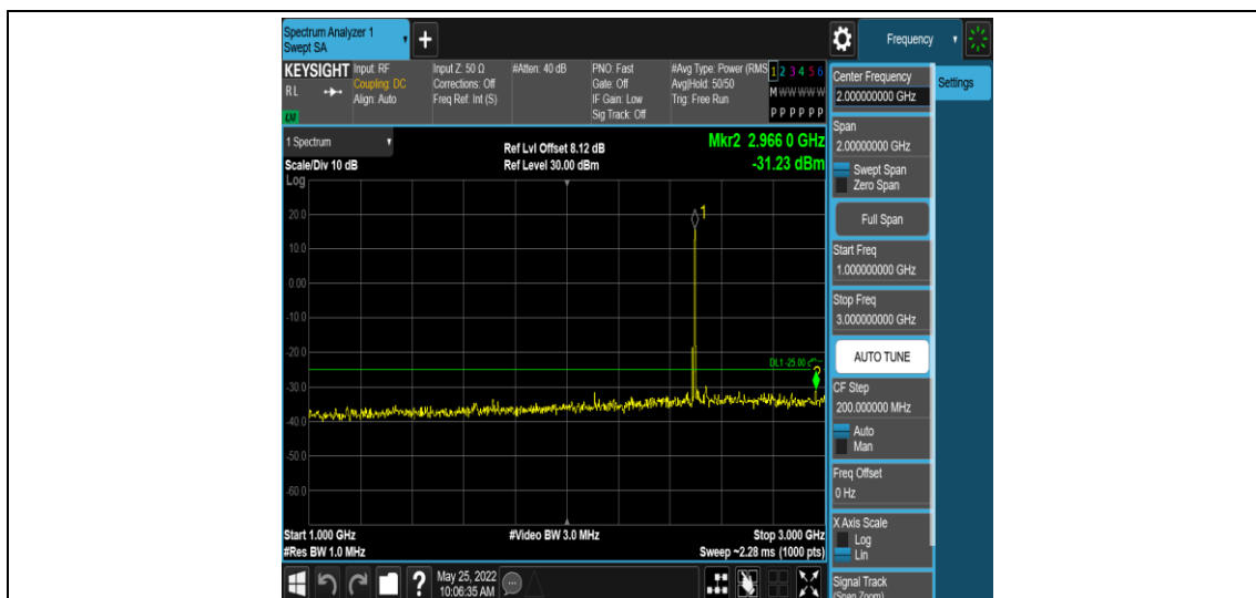
Band41-20MHz-QPSK-39750-1RB#0-Range4:1000~3000MHz
