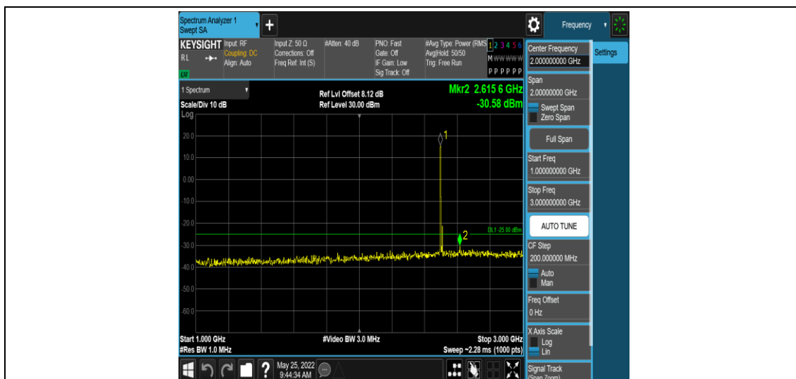
Band41-15MHz-QPSK-39725-1RB#0-Range4:1000~3000MHz
