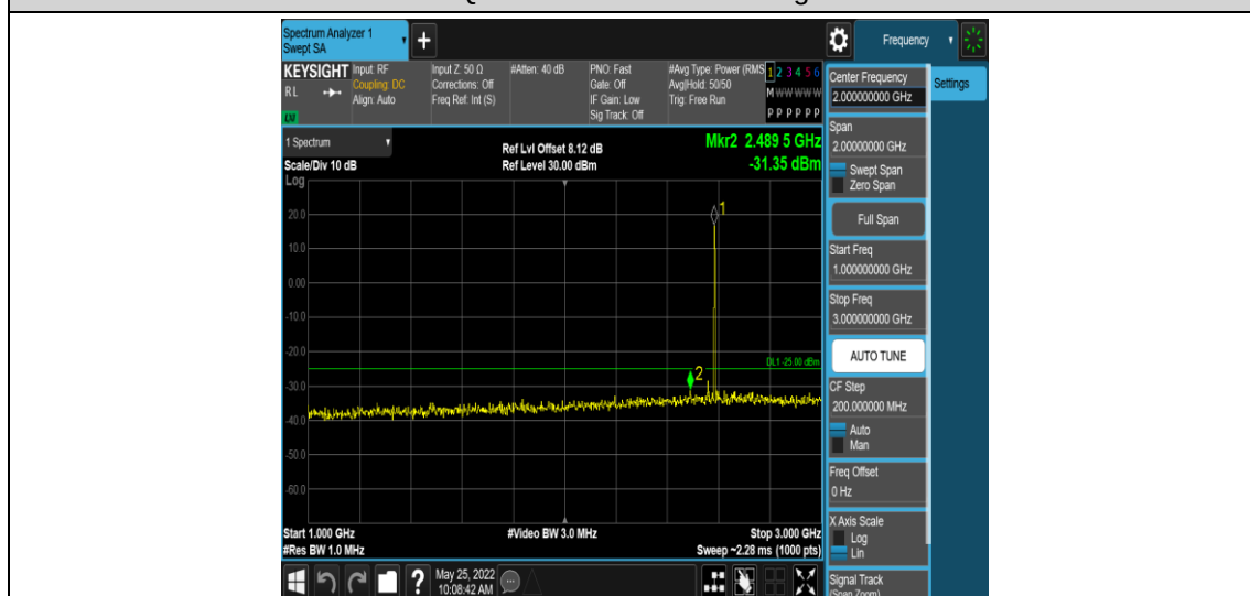
Band41-20MHz-QPSK-40620-1RB#0-Range4:1000~3000MHz
