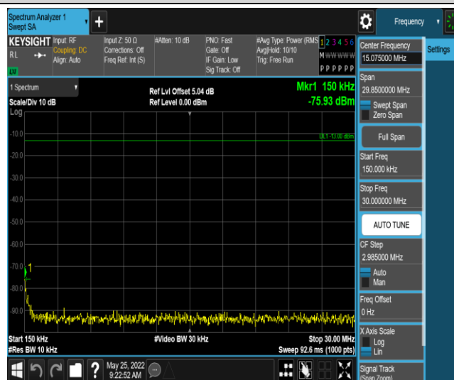
Band41-10MHz-QPSK-39700-1RB#0-Range2:0.15~30MHz
