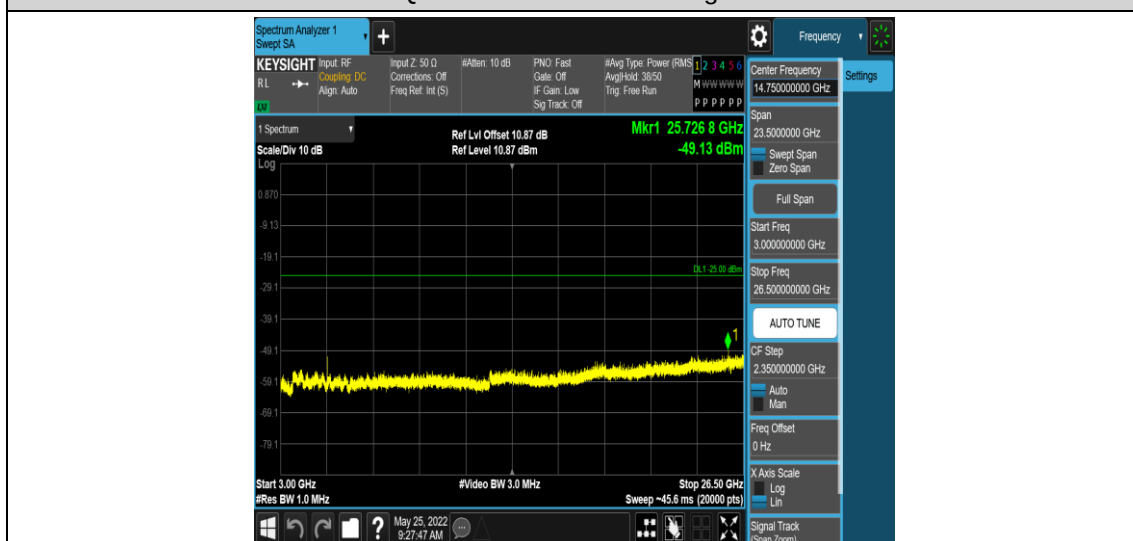
Band41-10MHz-QPSK-41540-1RB#0-Range5:3000~26500MHz
