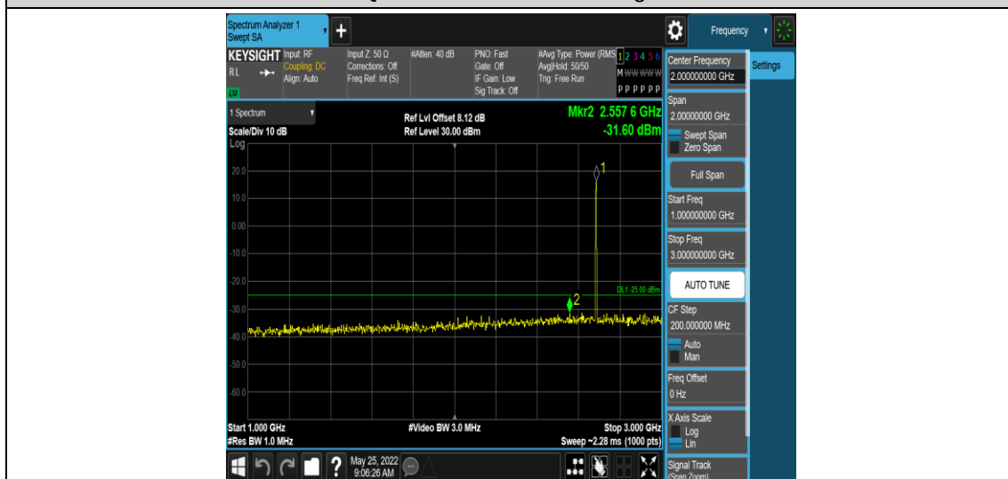
Band41-5MHz-QPSK-41565-1RB#0-Range4:1000~3000MHz
