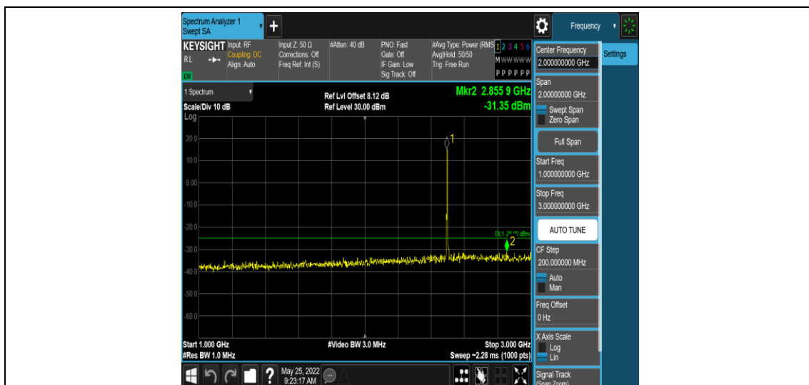
Band41-10MHz-QPSK-39700-1RB#0-Range4:1000~3000MHz
