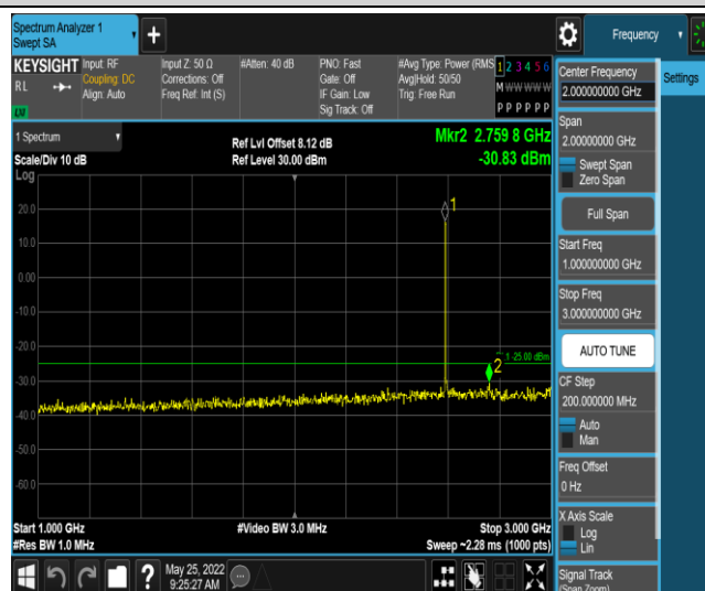
Band41-10MHz-QPSK-40620-1RB#0-Range4:1000~3000MHz
