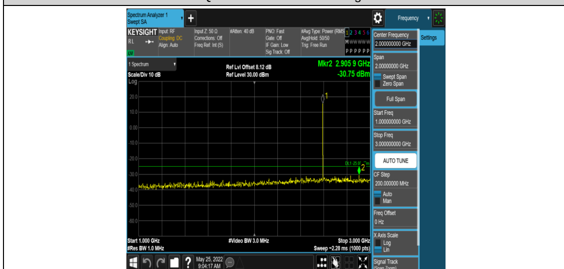
Band41-5MHz-QPSK-40620-1RB#0-Range4:1000~3000MHz
