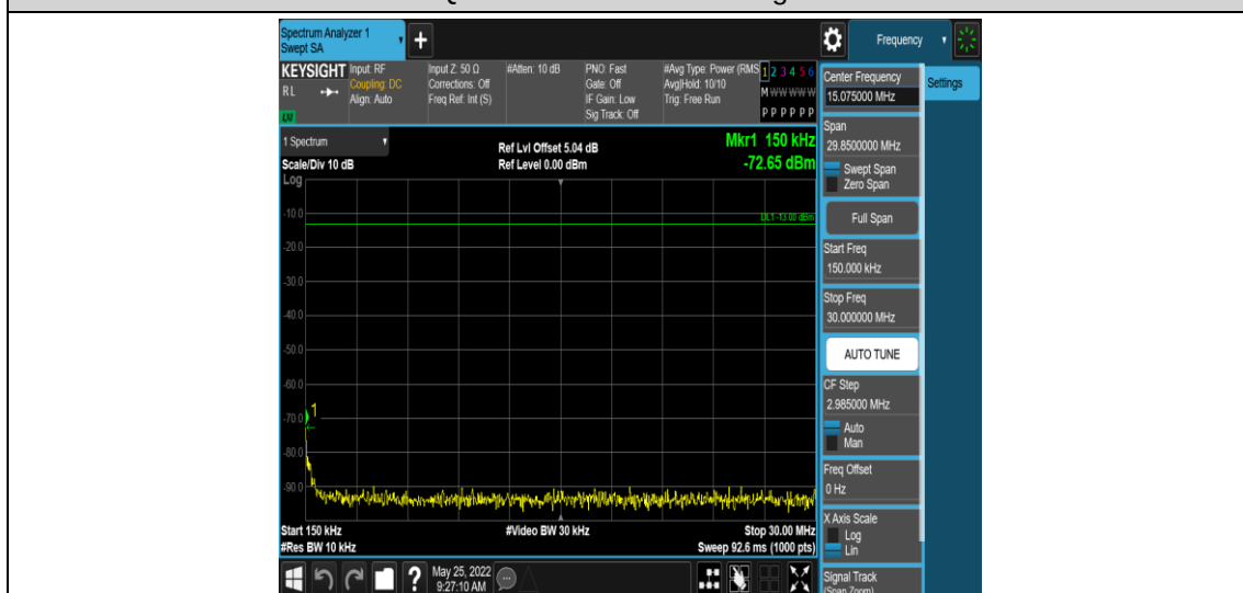
Band41-10MHz-QPSK-41540-1RB#0-Range2:0.15~30MHz
