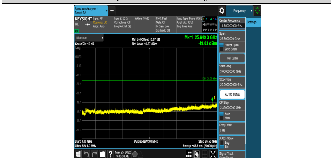
Band41-5MHz-QPSK-41565-1RB#0-Range5:3000~26500MHz
