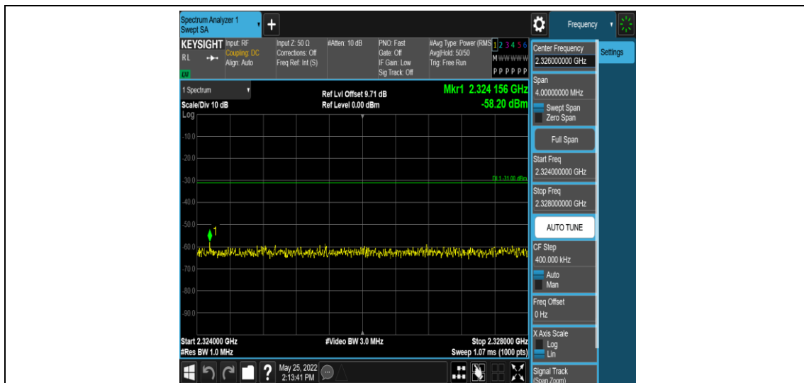
Band40-5MHz-QPSK-39225-1RB#0-Range10:2324~2328MHz
