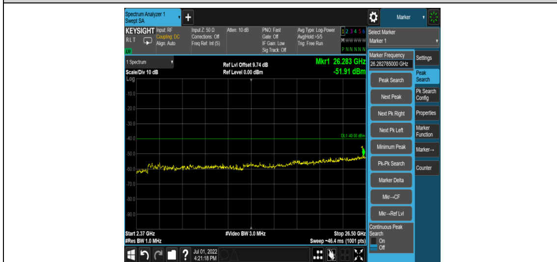
Band40-5MHz-QPSK-39225-1RB#0-Range15:2365~26500MHz
