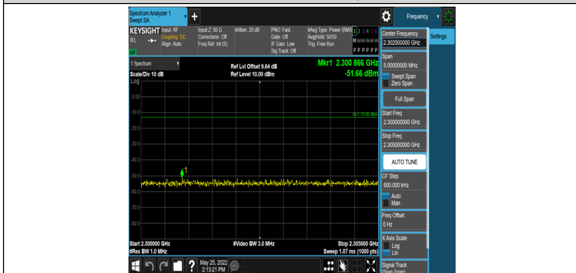
Band40-5MHz-QPSK-39225-1RB#0-Range8:2300~2305MHz
