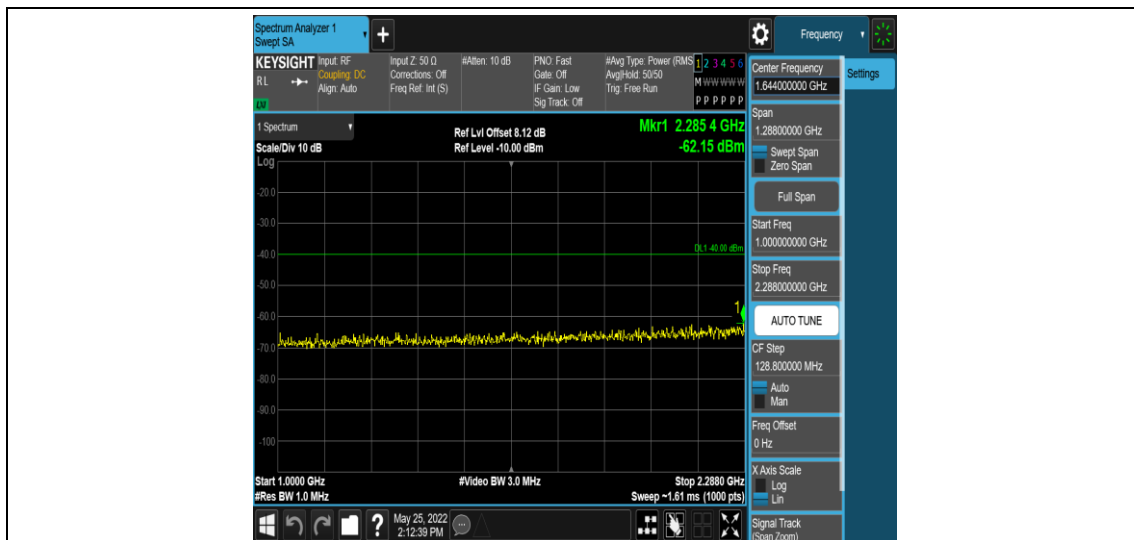
Band40-5MHz-QPSK-39225-1RB#0-Range4:1000~2288MHz
