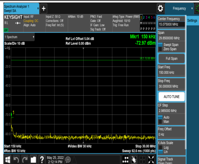
Band40-5MHz-QPSK-39225-1RB#0-Range2:0.15~30MHz
