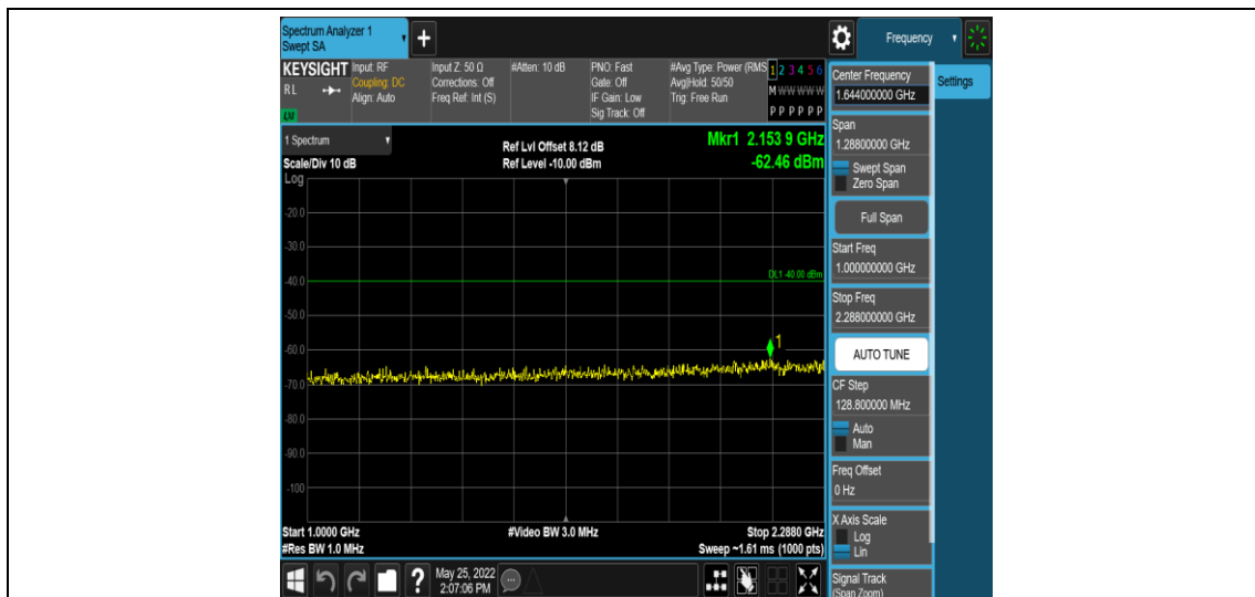
Band40-5MHz-QPSK-39200-1RB#0-Range4:1000~2288MHz
