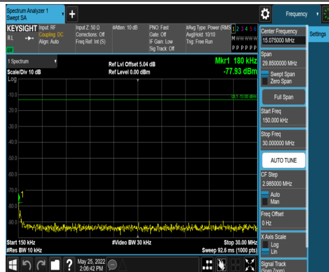
Band40-5MHz-QPSK-39200-1RB#0-Range2:0.15~30MHz
