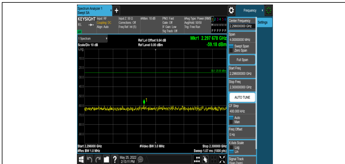
Band40-5MHz-QPSK-39225-1RB#0-Range7:2296~2300MHz
