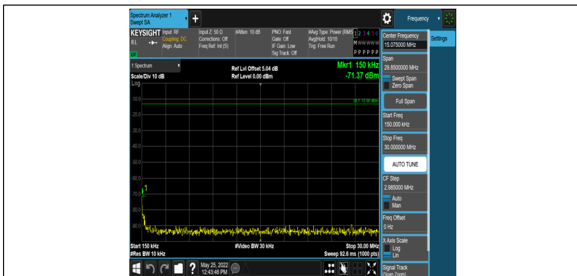
Band38-20MHz-QPSK-38150-1RB#0-Range2:0.15~30MHz
