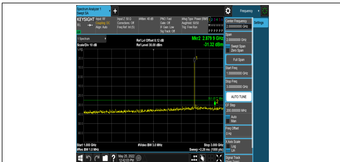
Band38-20MHz-QPSK-38000-1RB#0-Range4:1000~3000MHz
