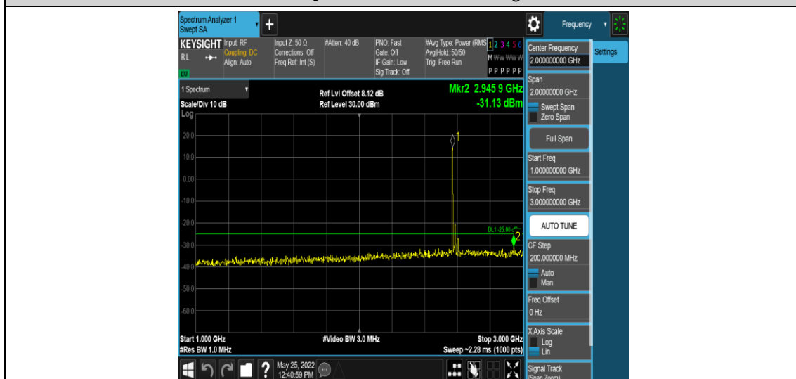
Band38-20MHz-16QAM-37850-1RB#0-Range4:1000~3000MHz
