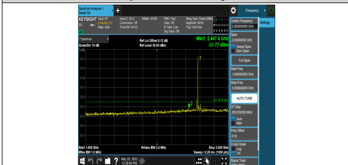
Band38-20MHz-QPSK-37850-1RB#0-Range4:1000~3000MHz
