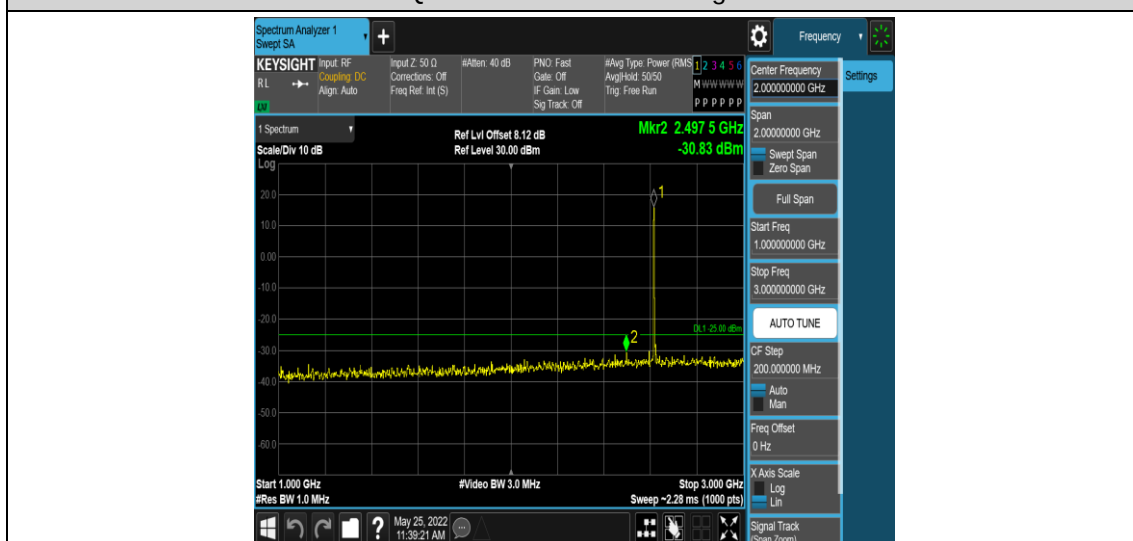
Band38-5MHz-QPSK-38225-1RB#0-Range4:1000~3000MHz
