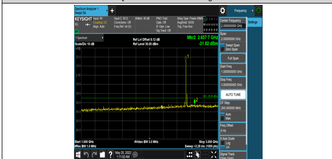
Band7-10MHz-QPSK-21100-1RB#0-Range4:1000~3000MHz
