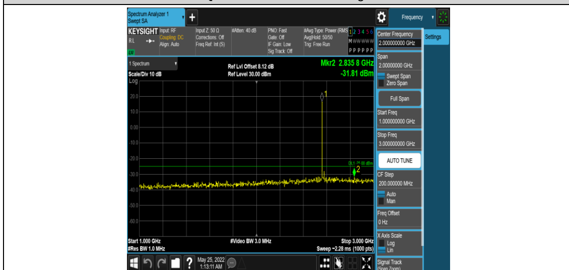
Band7-10MHz-QPSK-21400-1RB#0-Range4:1000~3000MHz
