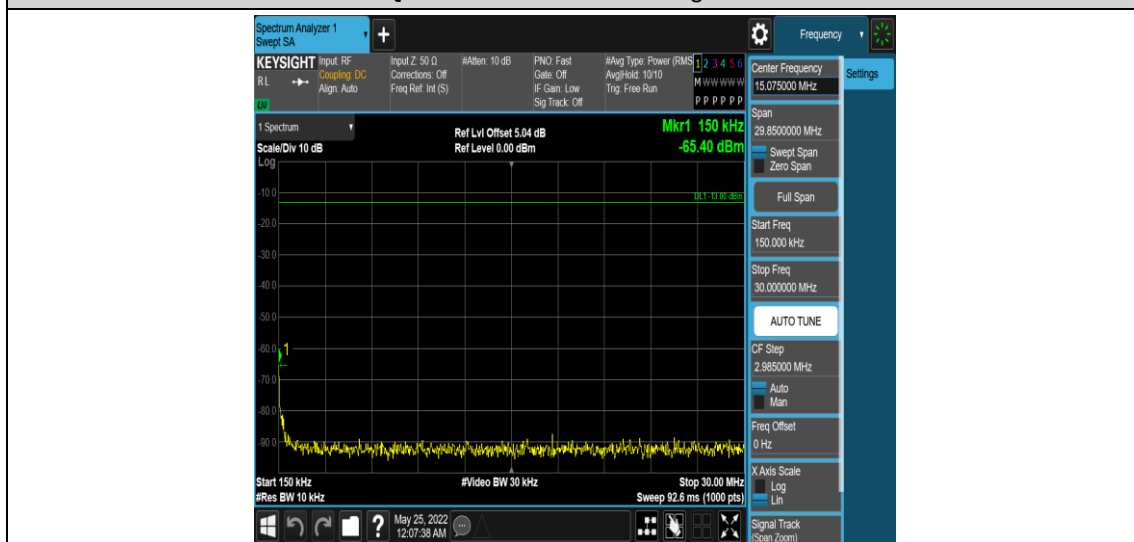
Band5-5MHz-QPSK-20425-1RB#0-Range2:0.15~30MHz
