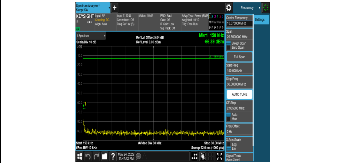
Band5-3MHz-QPSK-20415-1RB#0-Range2:0.15~30MHz
