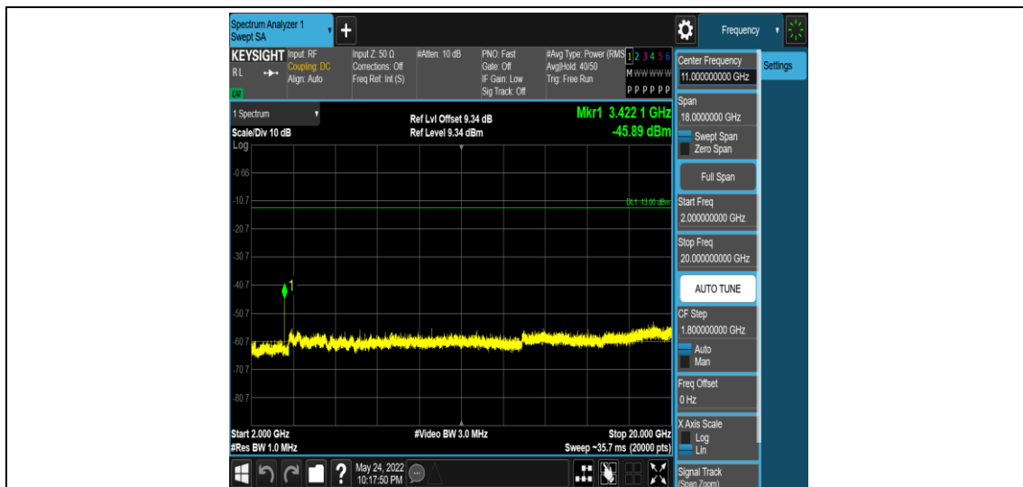
Band4-15MHz-QPSK-20025-1RB#0-Range5:2000~20000MHz
