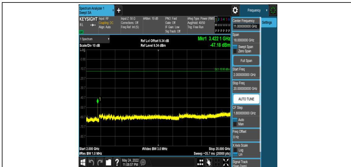
Band4-20MHz-QPSK-20050-1RB#0-Range5:2000~20000MHz
