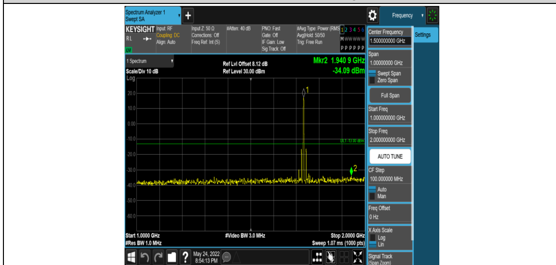
Band4-1.4MHz-QPSK-20175-1RB#0-Range4:1000~2000MHz
