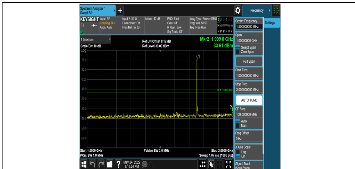
Band4-3MHz-QPSK-20385-1RB#0-Range4:1000~2000MHz
