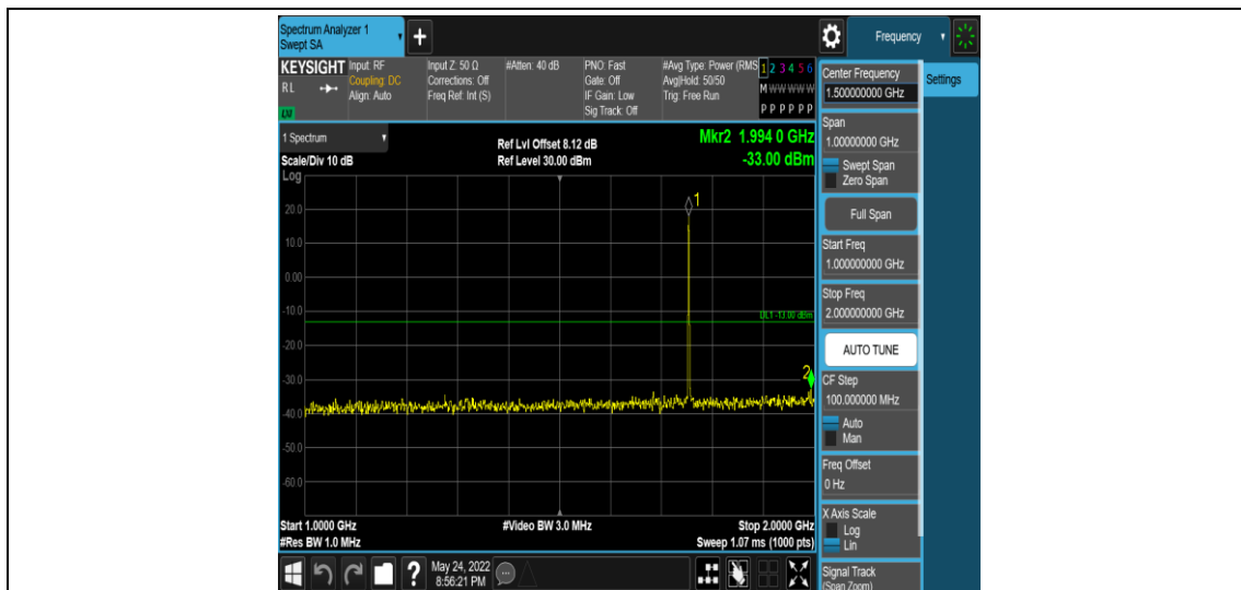
Band4-1.4MHz-QPSK-20393-1RB#0-Range4:1000~2000MHz
