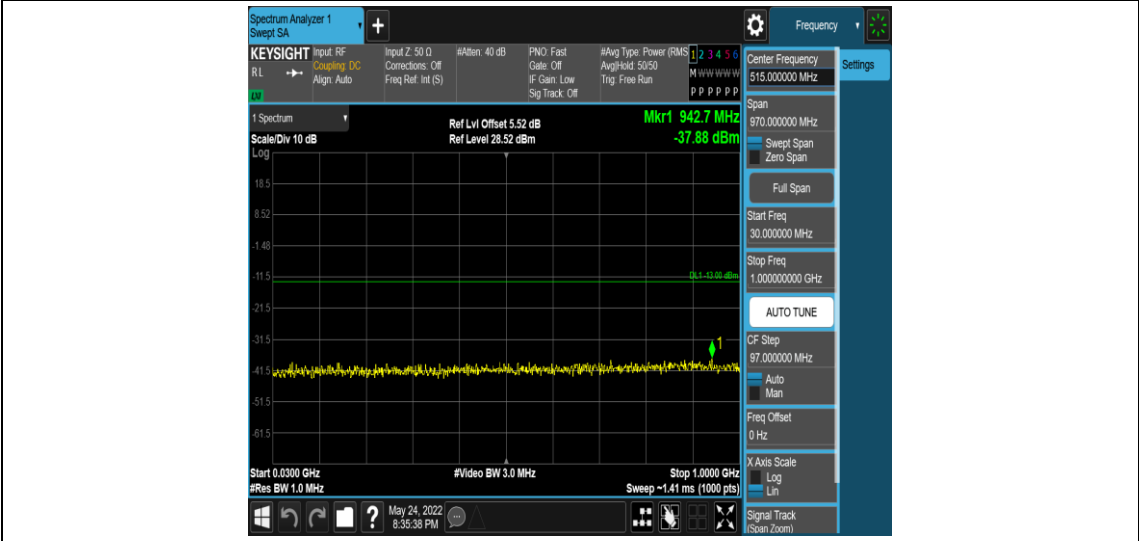
Band2-20MHz-QPSK-19100-1RB#0-Range3:30~1000MHz
