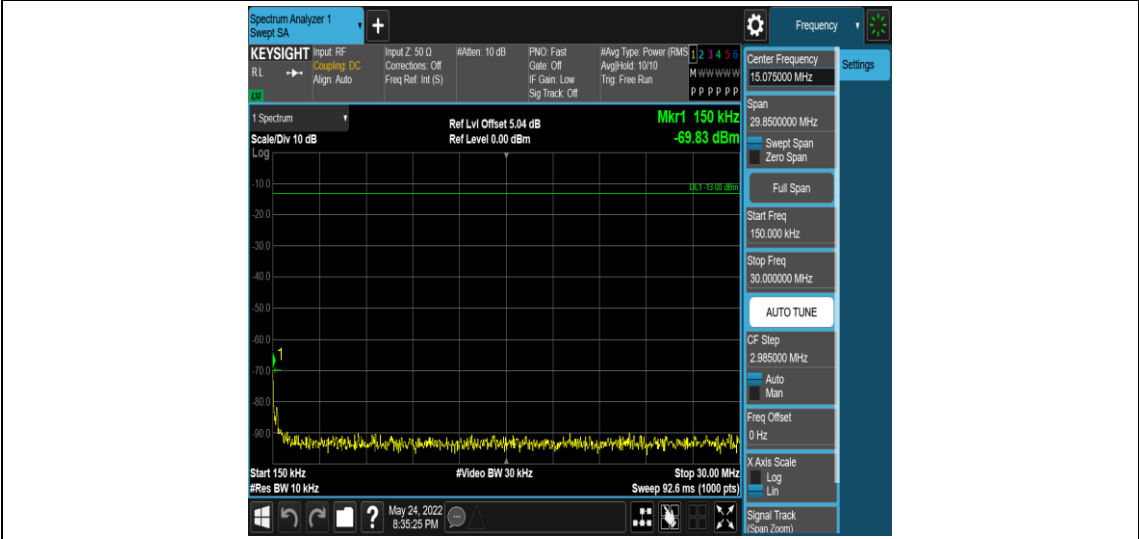
Band2-20MHz-QPSK-19100-1RB#0-Range2:0.15~30MHz
