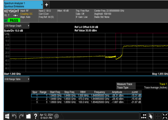
B66_N25(45M)_DFT-s- OFDM_BPSK_Outer_Full_Low_CH
