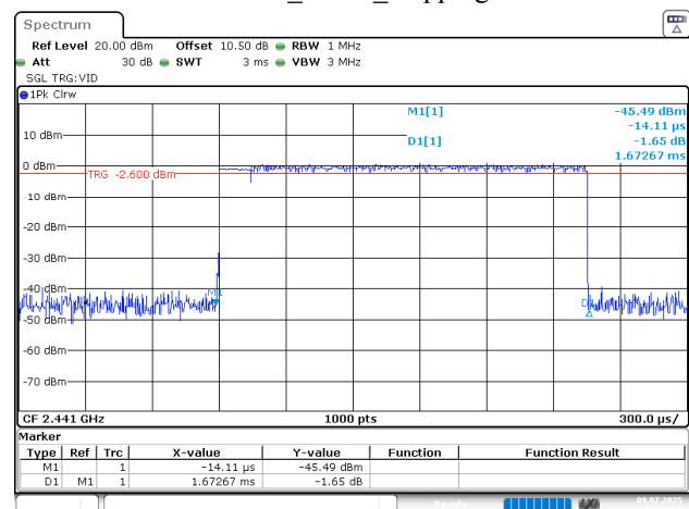
2EDR_2DH3_Hopping
