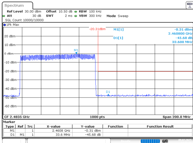
3EDR_DH1_Hopping_Upper
