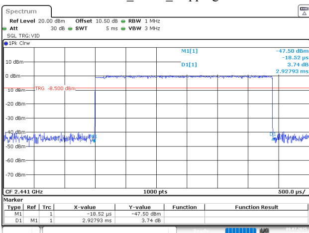
2EDR_2DH5_Hopping
