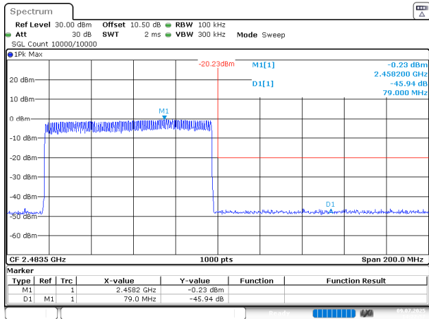
2EDR_DH1_Hopping_Upper
