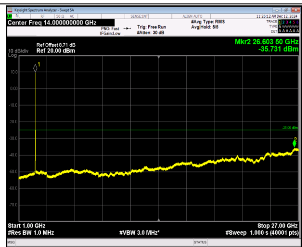
7-7-10MHz-20MHz-QPSK-QPSK-21206-21350-50RB#0-10 0RB#0-1000~27000MHz-PASS
