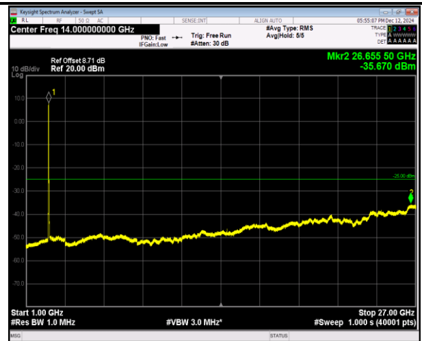
7-7-20MHz-10MHz-QPSK-QPSK-20850-20994-100RB#0-5 ORB#0-1000~27000MHz-PASS
