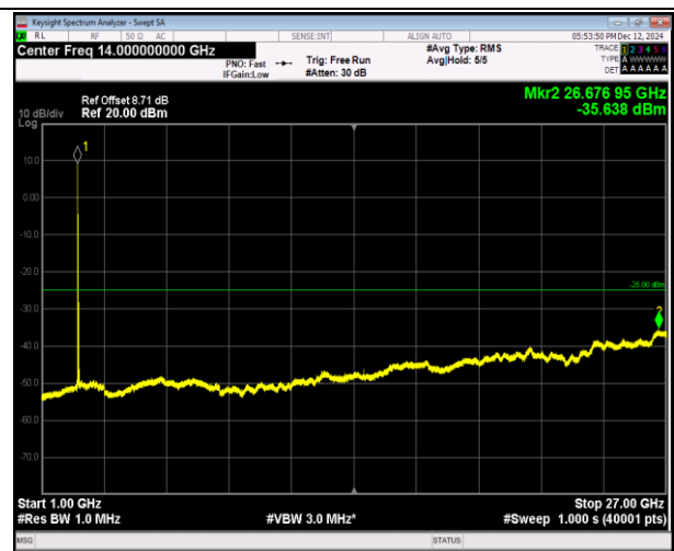
7-7-20MHz-10MHz-QPSK-QPSK-20850-20994-1RB#0-1RB #49-1000~27000MHz-PASS
