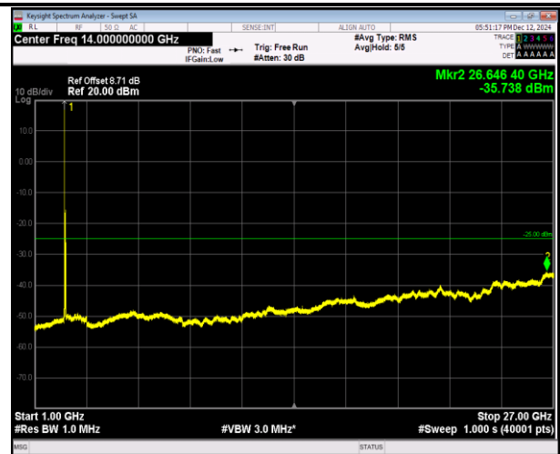
7-7-20MHz-10MHz-QPSK-QPSK-20850-20994-1RB#0-0RB #0-1000~27000MHz-PASS
