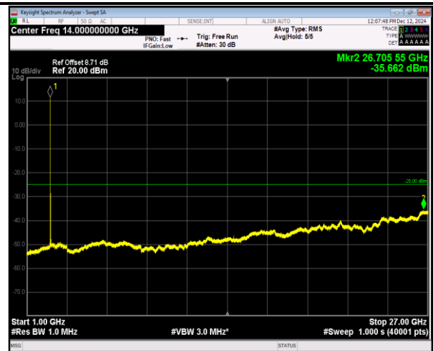
7-7-15MHz-10MHz-QPSK-QPSK-21051-21171-1RB#0-1RB #49-1000~27000MHz-PASS
