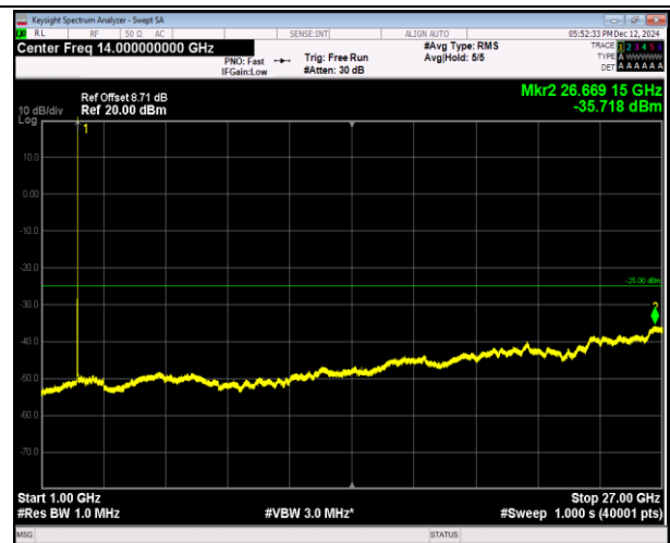
7-7-20MHz-10MHz-QPSK-QPSK-20850-20994-1RB#99-0R B#0-1000~27000MHz-PASS
