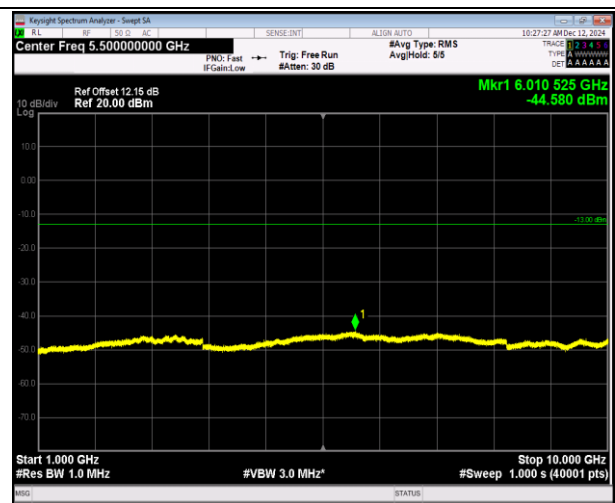
5-5-10MHz-10MHz-QPSK-QPSK-20501-20600-50RB#0-50 RB#0-1000~10000MHz-PASS
