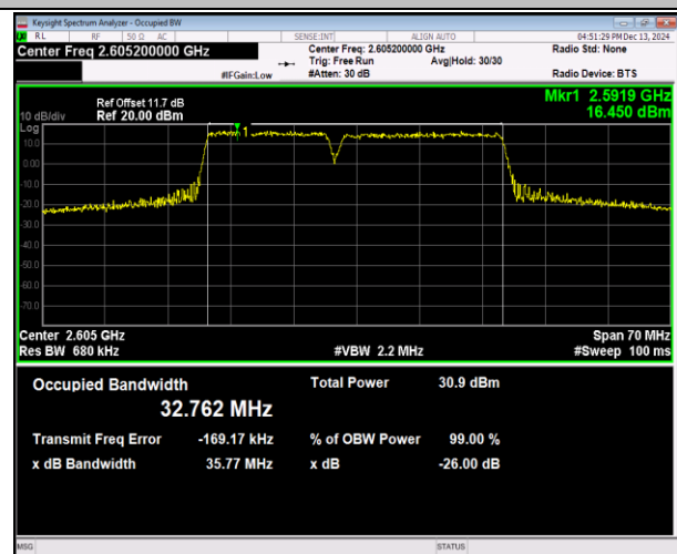
41(2555-2655)-41(2555-2655)-15MHz-20MHz-16QAM-16Q AM-40644-40815-75RB#0-100RB#0-PASS
