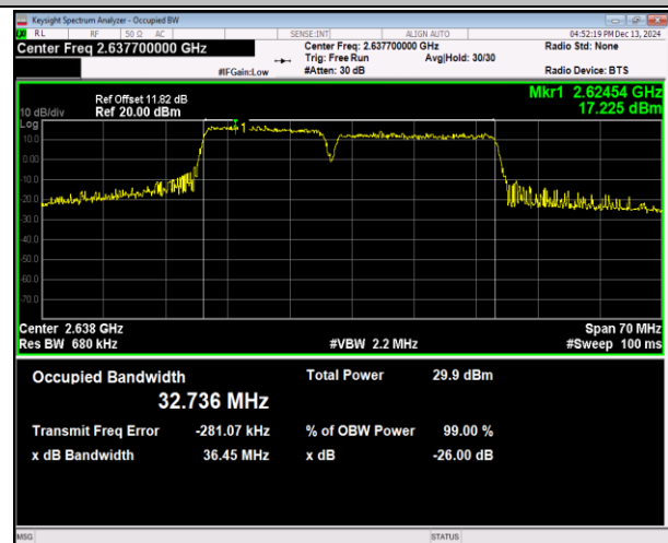
41(2555-2655)-41(2555-2655)-15MHz-20MHz-16QAM-16Q AM-40969-41140-75RB#0-100RB#0-PASS
