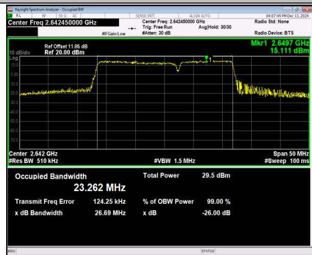
41(2555-2655)-41(2555-2655)-15MHz-10MHz-16QAM-16Q AM-41067-41187-75RB#0-50RB#0-PASS
