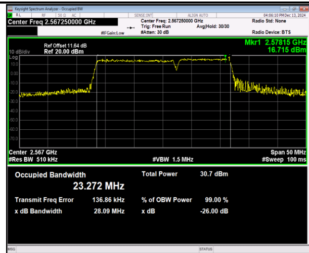
41(2555-2655)-41(2555-2655)-15MHz-10MHz-16QAM-16Q AM-40315-40435-75RB#0-50RB#0-PASS
