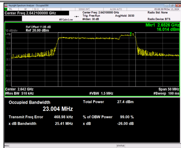
41(2555-2655)-41(2555-2655)-20MHz-5MHz-16QAM-16QA M-41090-41207-100RB#0-25RB#0-PASS
