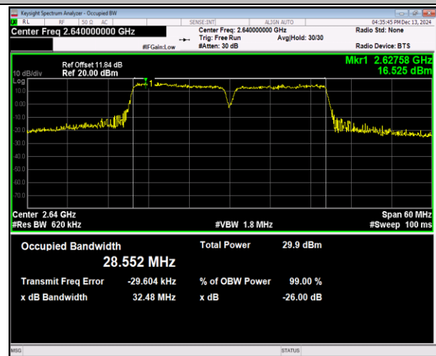
41(2555-2655)-41(2555-2655)-15MHz-15MHz-16QAM-16Q AM-41015-41165-75RB#0-75RB#0-PASS
