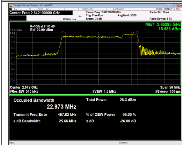
41(2555-2655)-41(2555-2655)-20MHz-5MHz-QPSK-QPS K-41090-41207-100RB#0-25RB#0-PASS
