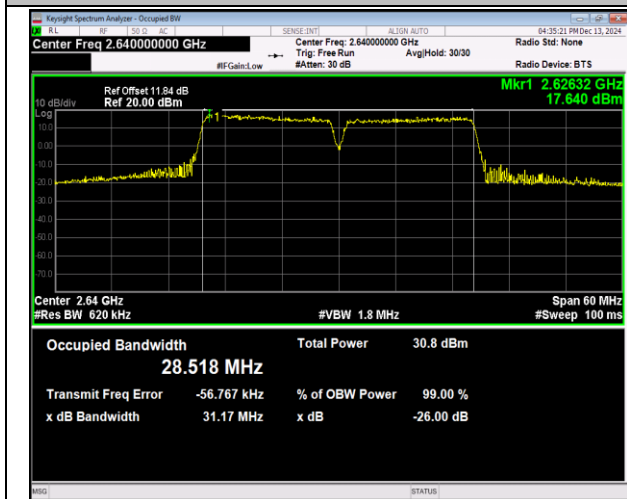
41(2555-2655)-41(2555-2655)-15MHz-15MHz-QPSK-QP SK-41015-41165-75RB#0-75RB#0-PASS
