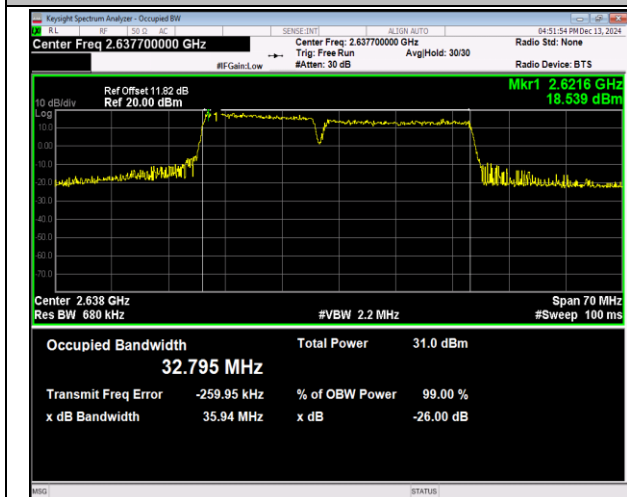
41(2555-2655)-41(2555-2655)-15MHz-20MHz-QPSK-QP SK-40969-41140-75RB#0-100RB#0-PASS
