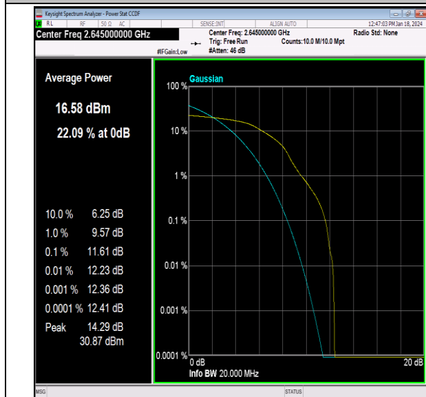
41(2535-2655)-20MHz-16QAM-41140-1RB#0-PASS
