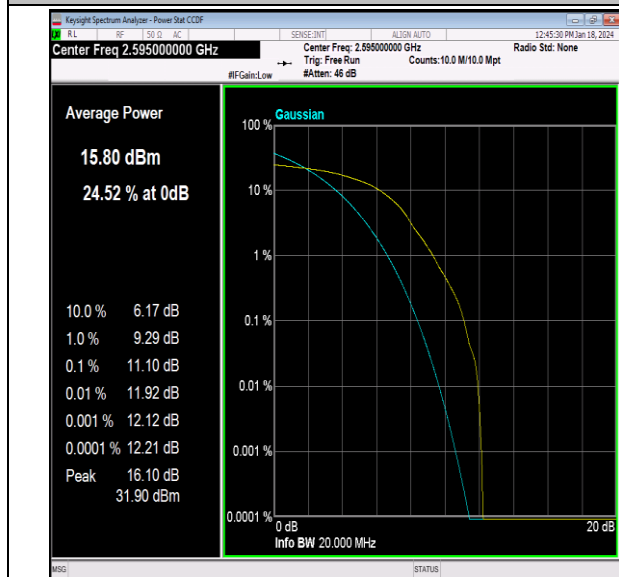
41(2535-2655)-20MHz-64QAM-40640-1RB#0-PASS
