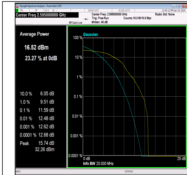
41(2535-2655)-20MHz-16QAM-40640-1RB#0-PASS
