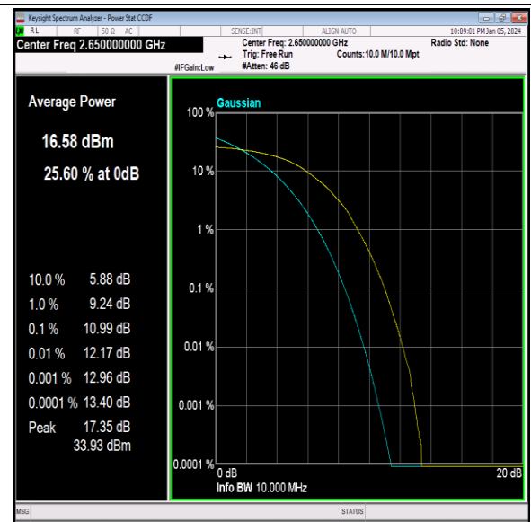
41(2535-2655)-10MHz-64QAM-41190-50RB#0-PASS
