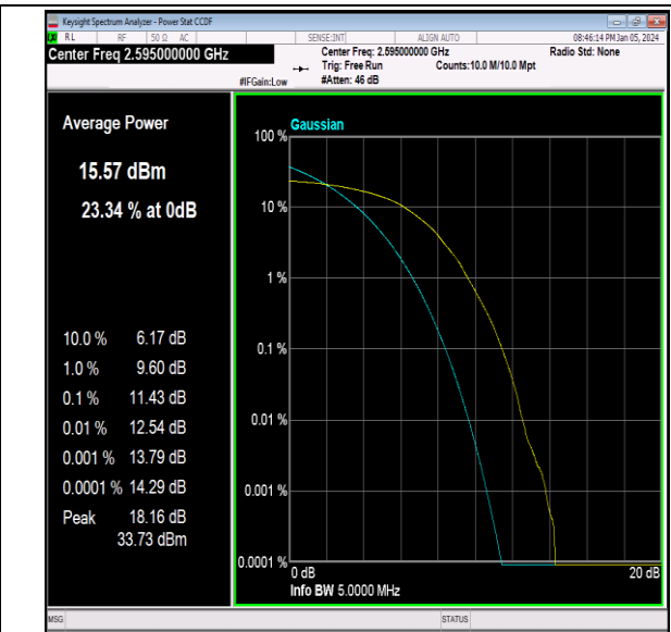
41(2535-2655)-5MHz-64QAM-40640-25RB#0-PASS
