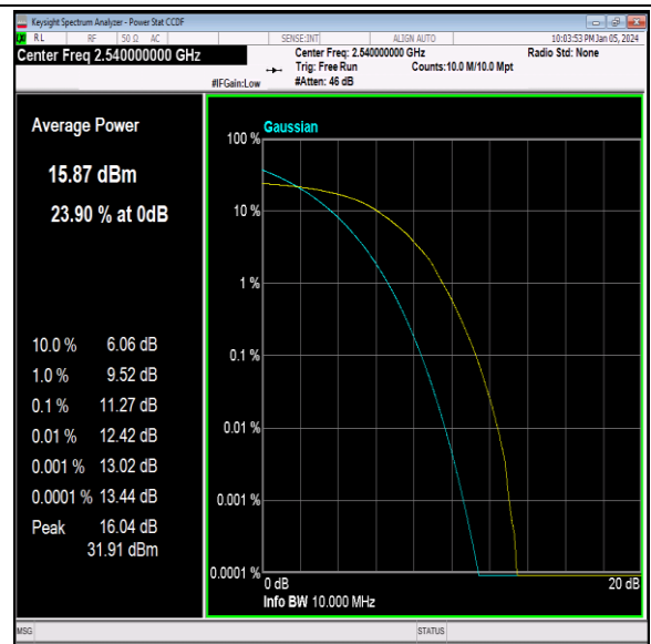
41(2535-2655)-10MHz-64QAM-40090-50RB#0-PASS
