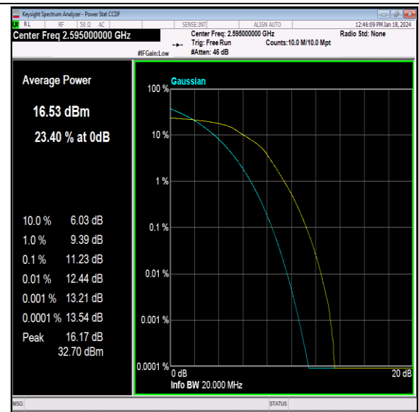
41(2535-2655)-20MHz-16QAM-40640-100RB#0-PASS
