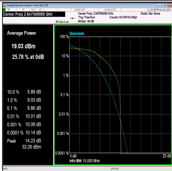
41(2535-2655)-15MHz-QPSK-41165-1RB#0-PASS
