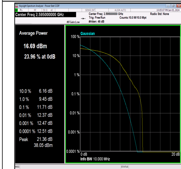
41(2535-2655)-10MHz-64QAM-40640-1RB#0-PASS
