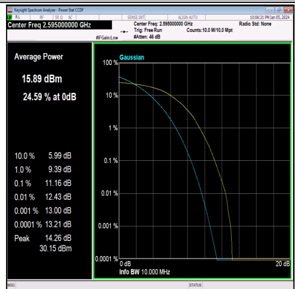
41(2535-2655)-10MHz-64QAM-40640-50RB#0-PASS
