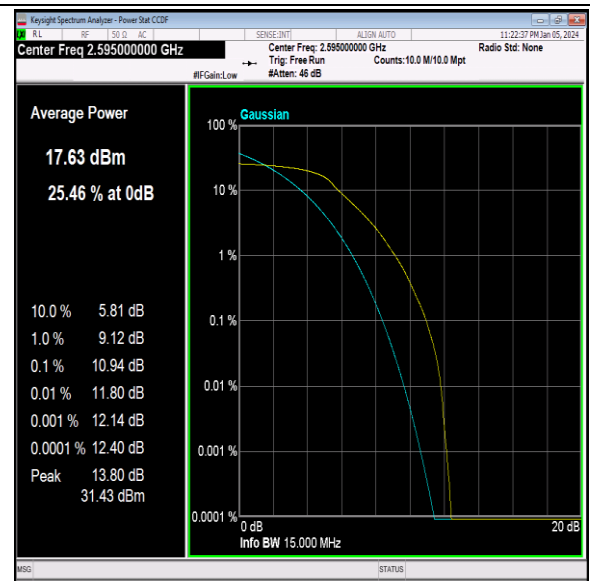
41(2535-2655)-15MHz-QPSK-40640-75RB#0-PASS
