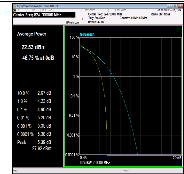
26(824-849)-1.4MHz-QPSK-26797-6RB#0-PASS
