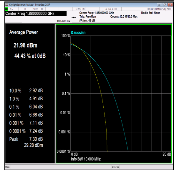
Band2-10MHz-16QAM-18900-50RB#0-PASS
