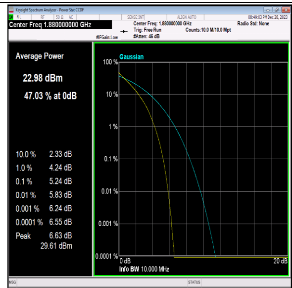
Band2-10MHz-QPSK-18900-50RB#0-PASS
