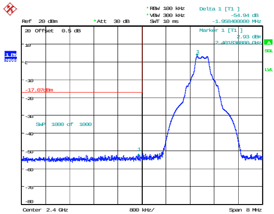
DH1_Low 54.94dB
