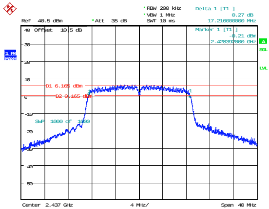
802.11n20_2437MHz
