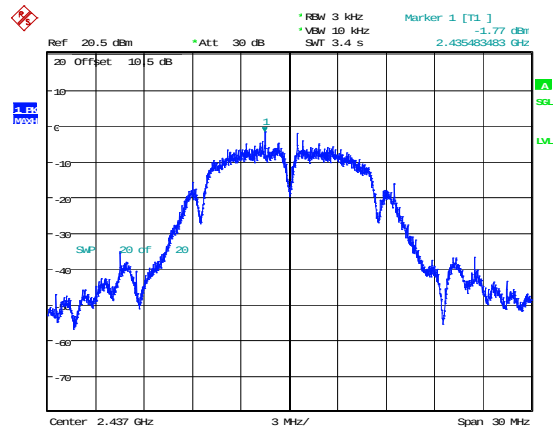
802.11b_2437MHz
