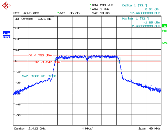
802.11n20_2412MHz
