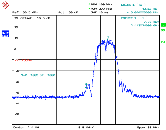
802.11b_2412MHz
