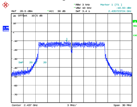
802.11g_2437MHz
