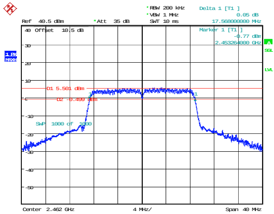
802.11n20_2462MHz
