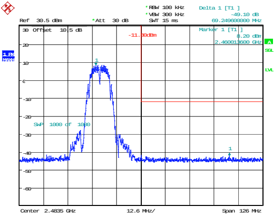
802.11b_2462MHz
