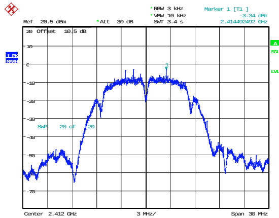
802.11b_2412MHz
