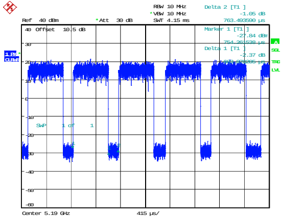
802.11ac40_5190MHz
