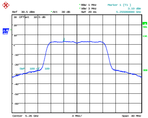
802.11n20_5260MHz
