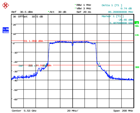
802.11ac80_5530MHz
