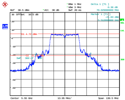
802.11ac40_5550MHz
