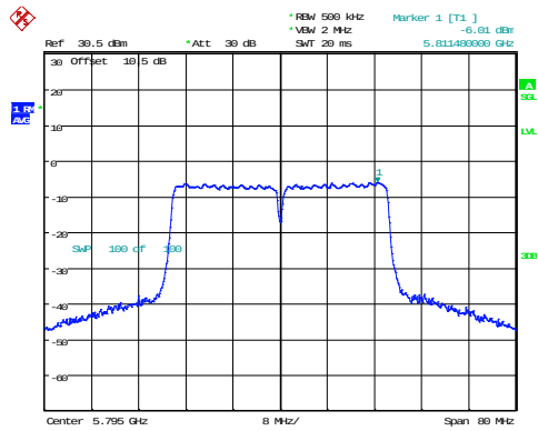
802.11ac40_5795MHz
