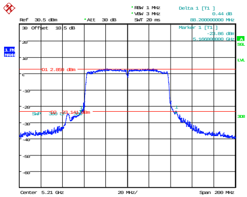
802.11ac80_5210MHz
