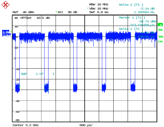
802.11n20_5200MHz
