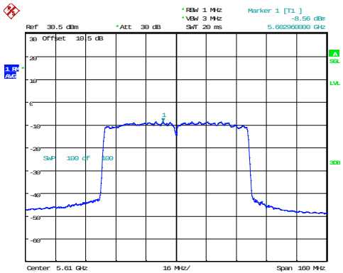
802.11ac80_5610MHz
