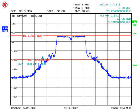
802.11ac40_5230MHz
