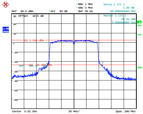
802.11ac80_5610MHz
