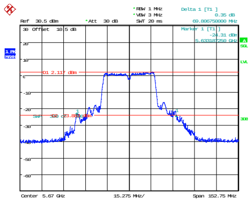
802.11ac40_5670MHz
