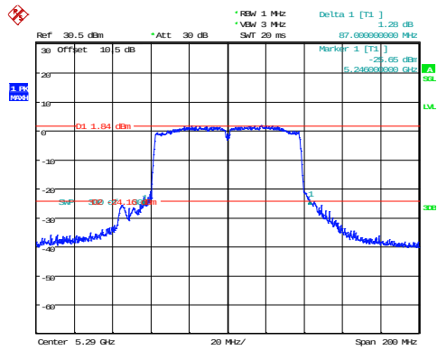
802.11ac80_5290MHz
