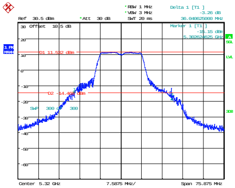
802.11a_5320MHz
