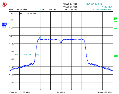
802.11ac40_5230MHz
