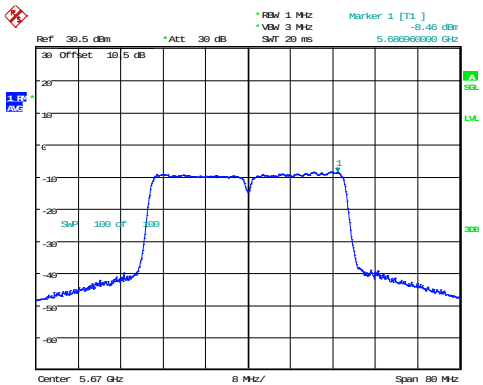
802.11ac40_5670MHz
