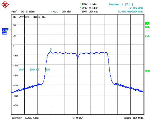
802.11ac40_5510MHz
