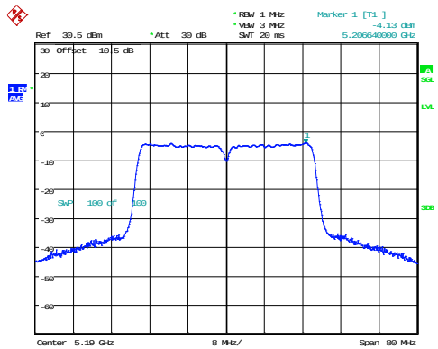
802.11ac40_5190MHz
