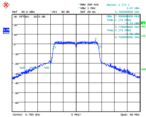
802.11n20_5785MHz
