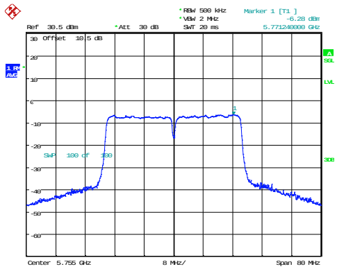
802.11ac40_5755MHz
