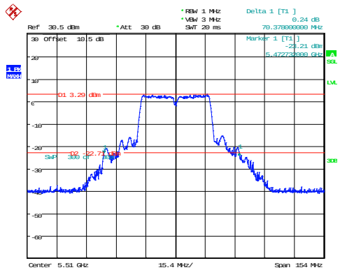
802.11ac40_5510MHz
