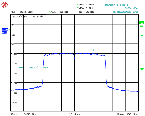
802.11ac80_5530MHz
