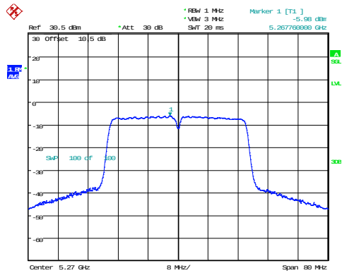
802.11ac40_5270MHz
