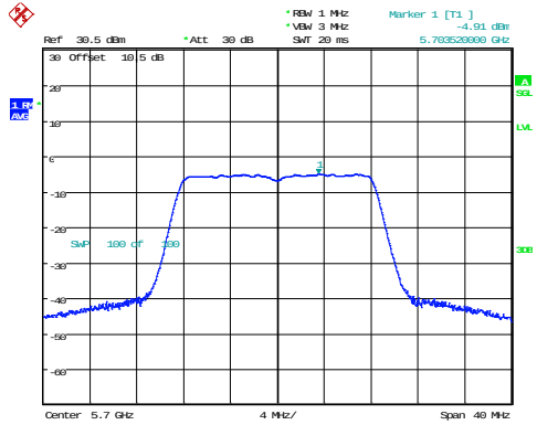
802.11a_5700MHz
