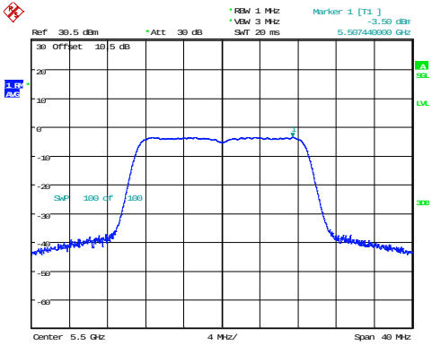
802.11n20_5500MHz
