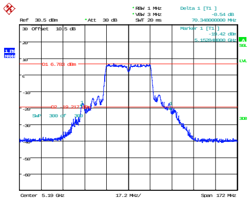
802.11ac40_5190MHz
