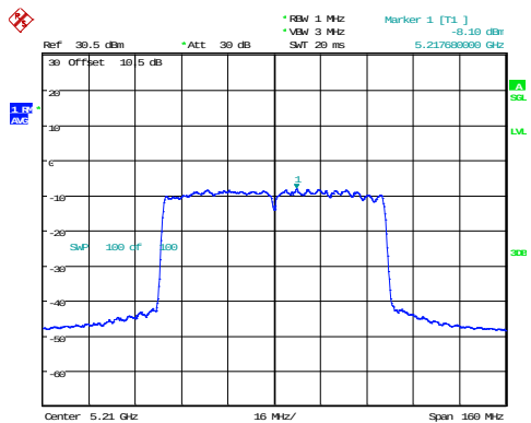
802.11ac80_5210MHz
