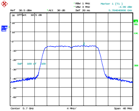
802.11n20_5700MHz
