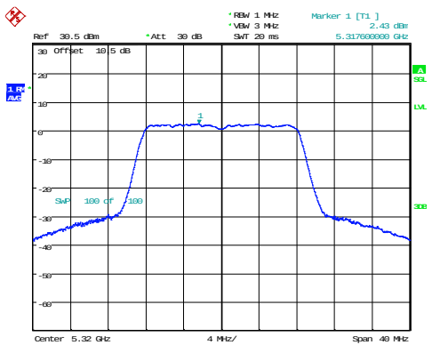
802.11a_5320MHz
