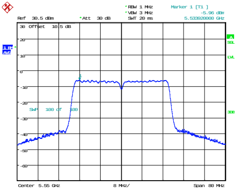
802.11ac40_5550MHz
