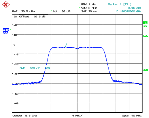
802.11a_5500MHz
