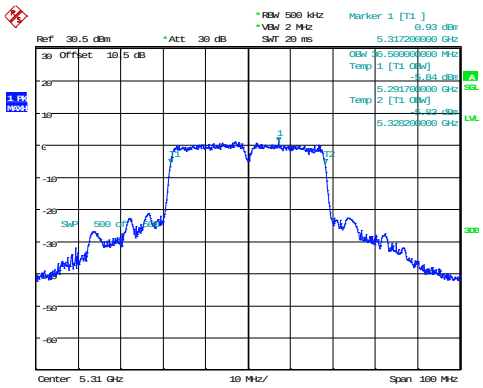
802.11ac40_5310MHz
