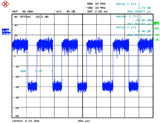
802.11ac80_5210MHz
