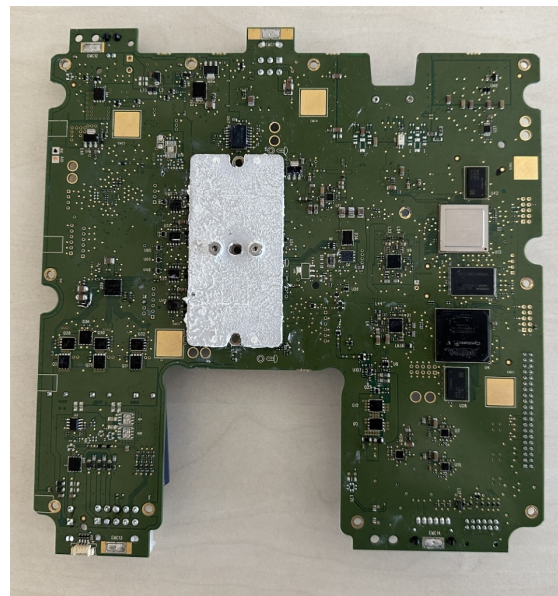
CPU PCBA - Bottom
