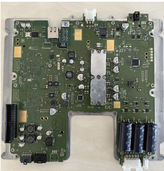
CPU PCBA - Top
