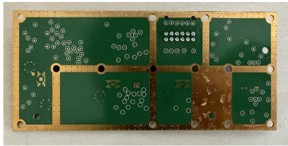
PM Module PCBA - Bottom
