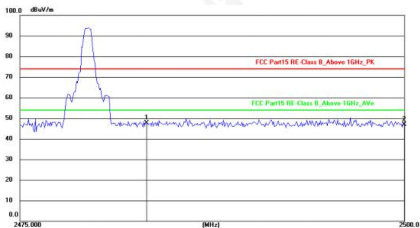
2480MHz Horizontal
