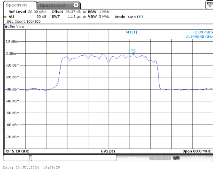
11N40MIMO_Ant2_5190
