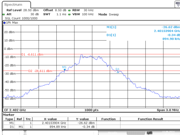
GFSK_Low 0.895MHz
