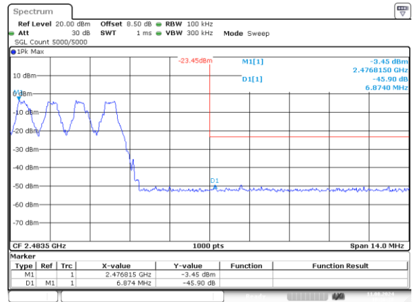
GFSK_Hopping_Upper 45.90dB
