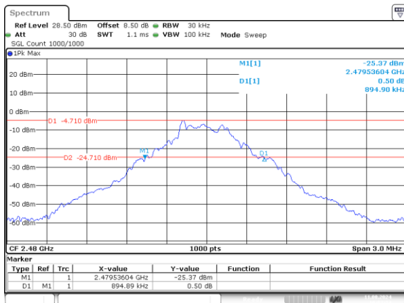
GFSK_High 0.895MHz
