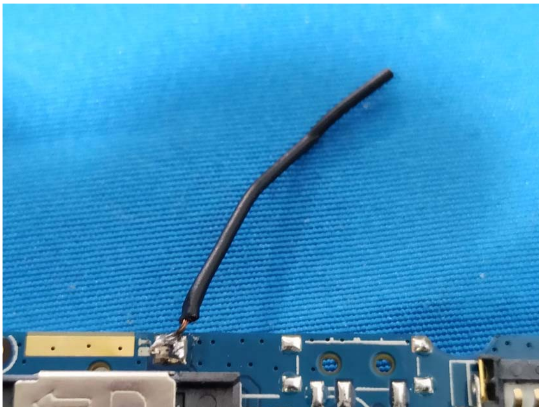
GSM ANT
