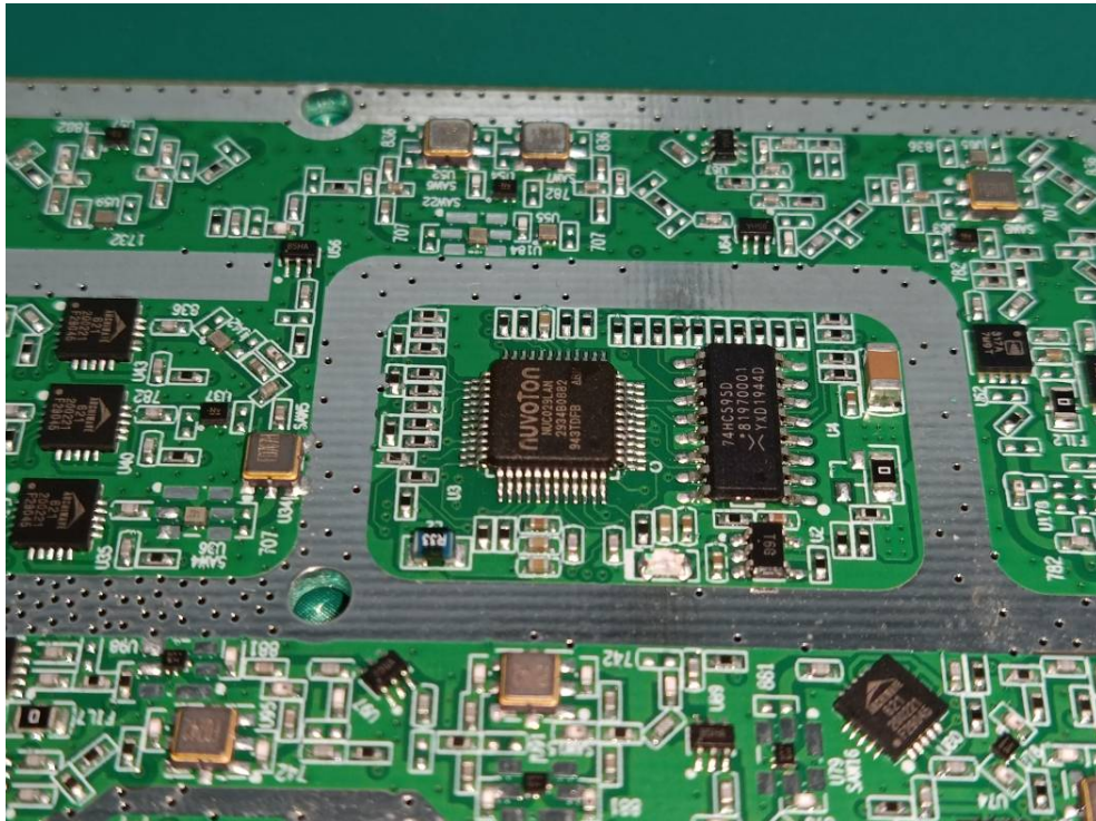
Wi-Fi Module
