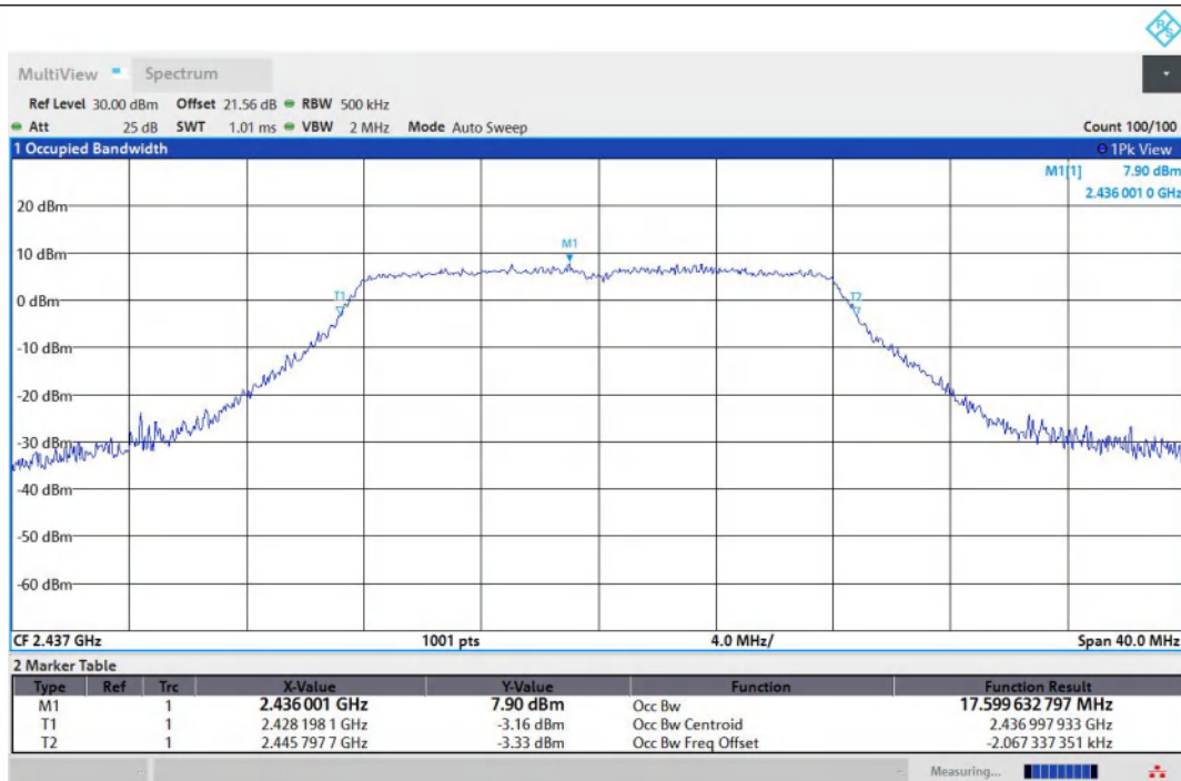
11G-Ant1-2437
