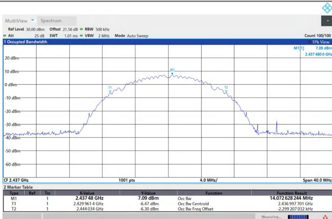
11B-Ant1-2437
