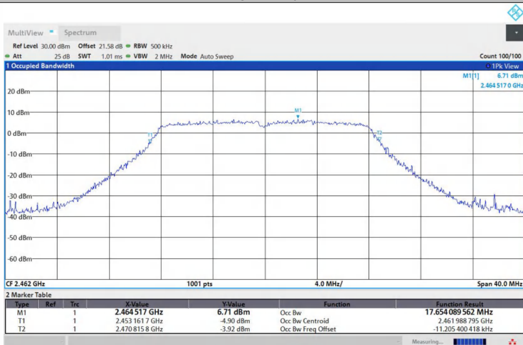
11G-Ant1-2462
