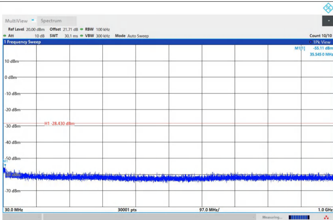
11G-Ant1-2412-30~1000-PASS
