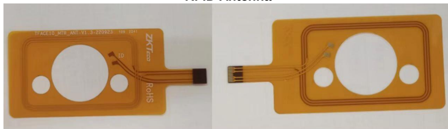
RFID Antenna
