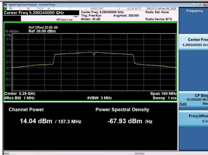
11AC80SISO-Ant1-5290-PASS
