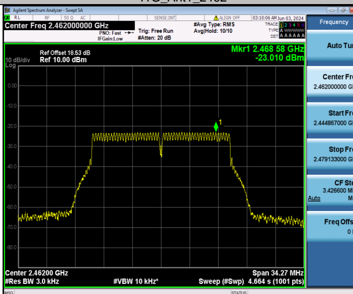
11G_Ant1_2462
