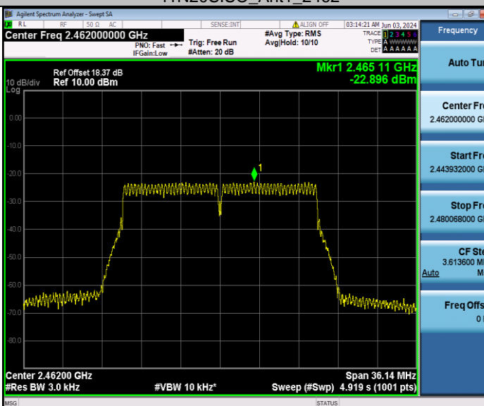
11N20SISO_Ant1_2462
