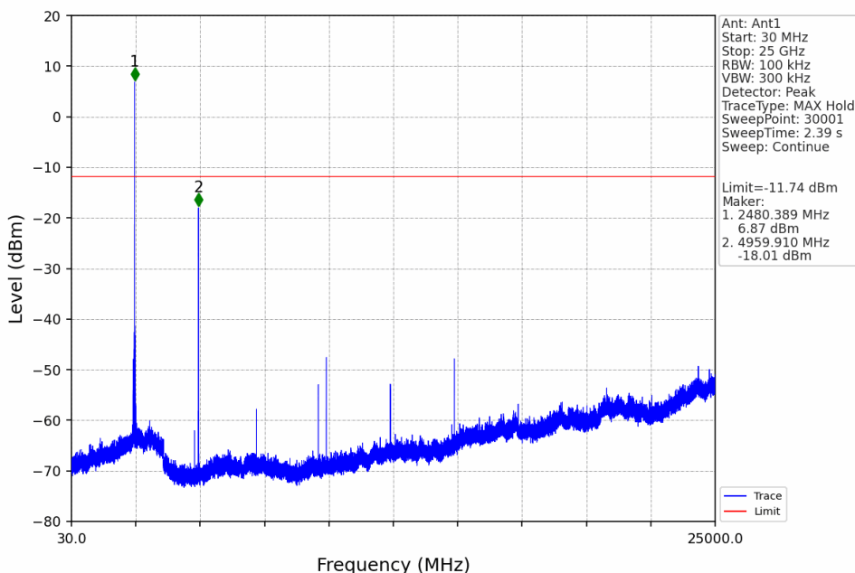
1M_HOPP_Ant1_NTNV
