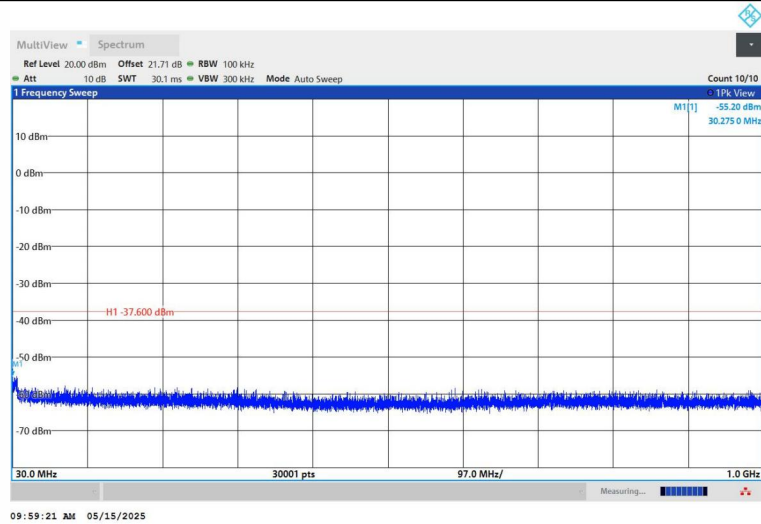
11G-Ant1-2412-30~1000-PASS
