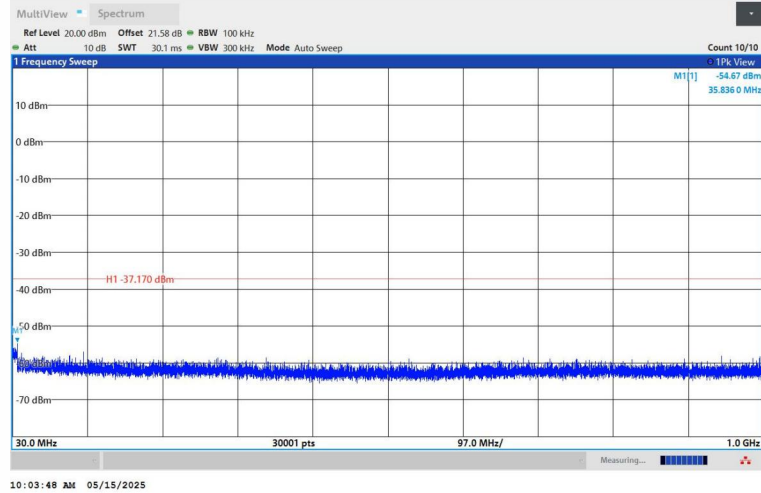
11G-Ant1-2462-30~1000-PASS
