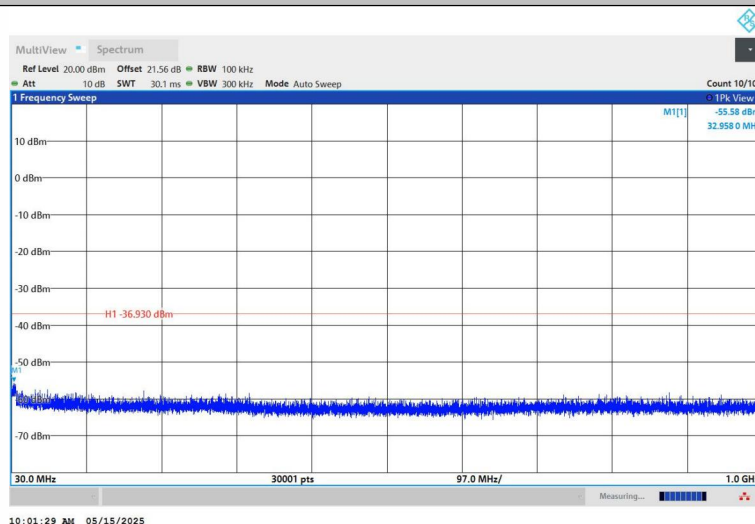
11G-Ant1-2437-30~1000-PASS
