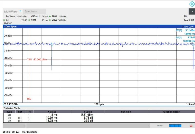
NTNV-11G-Ant1-2437
