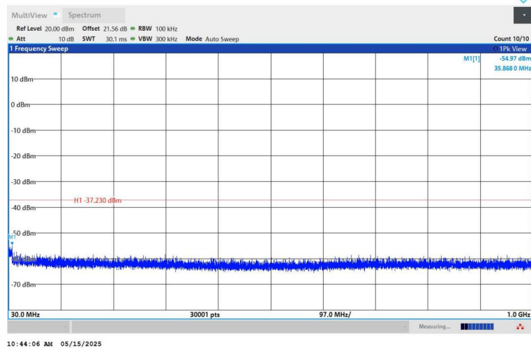
11G-Ant1-2437-30~1000-PASS
