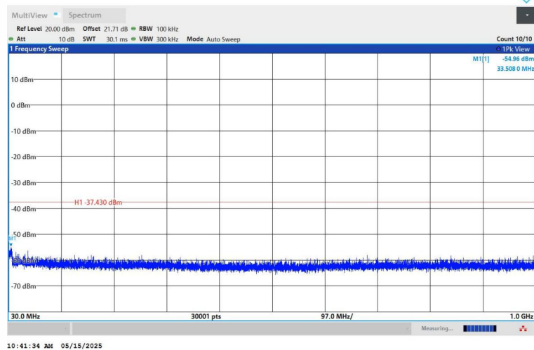
11G-Ant1-2412-30~1000-PASS
