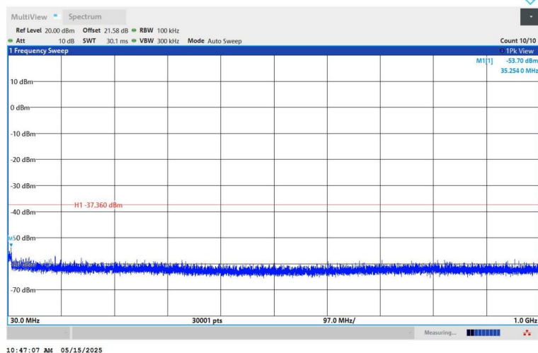
11G-Ant1-2462-30~1000-PASS
