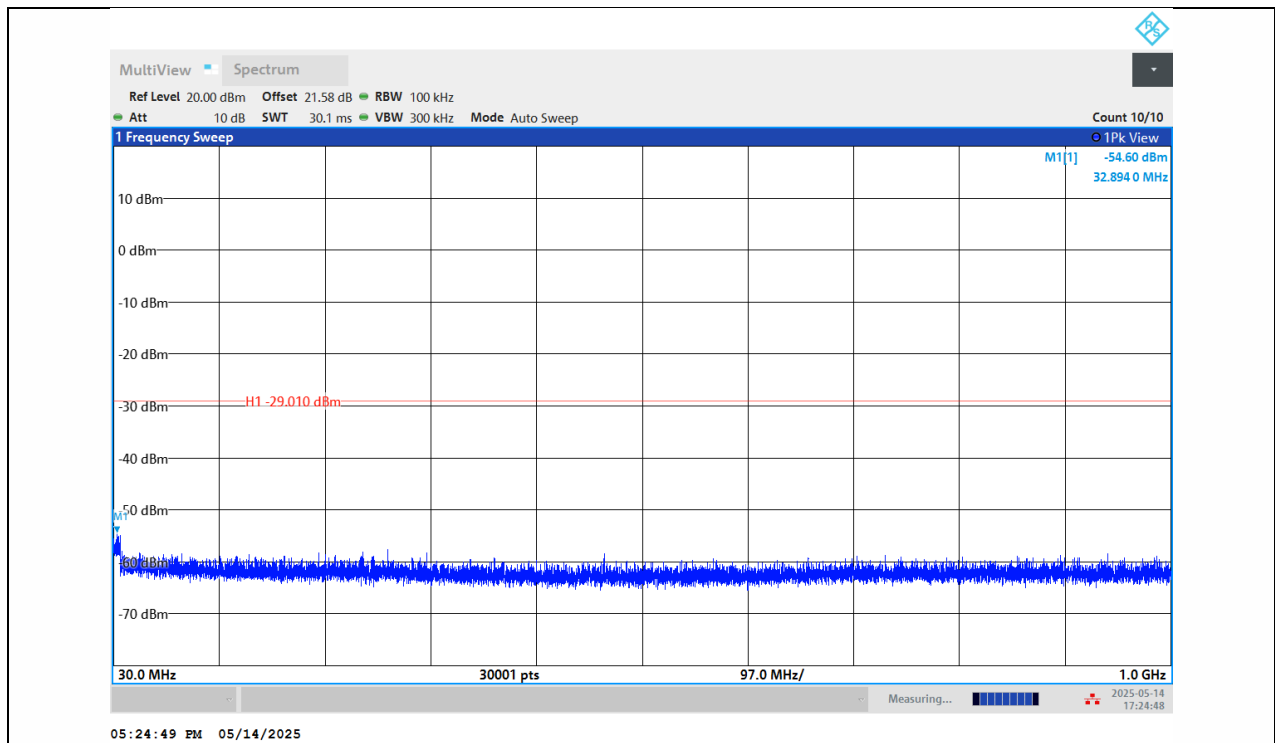
11G-Ant1-2462-30~1000-PASS
