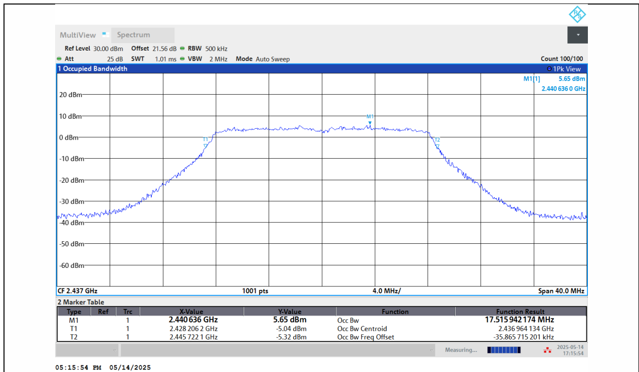
11G-Ant1-2437
