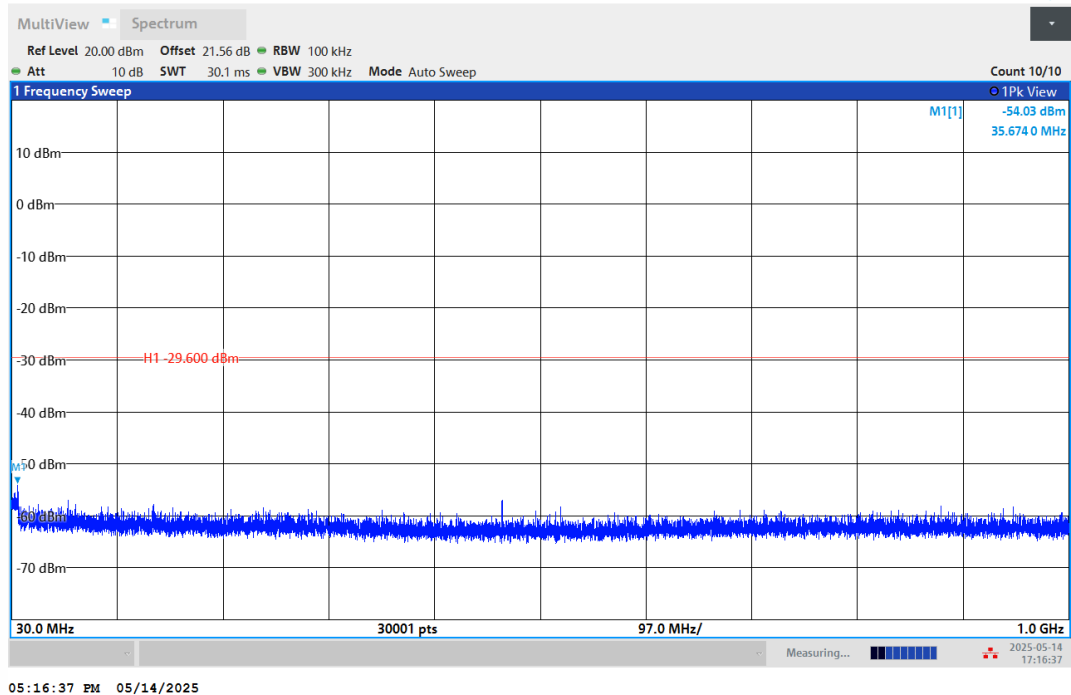
11G-Ant1-2437-30~1000-PASS
