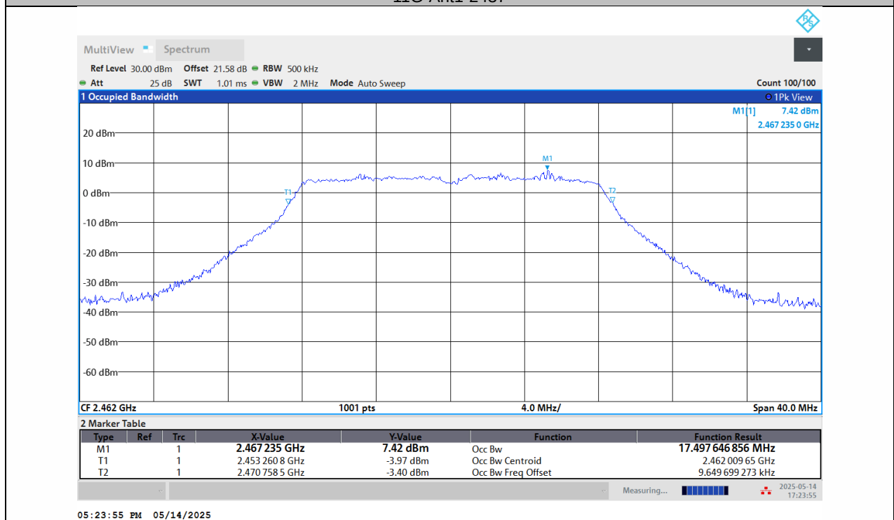
11G-Ant1-2462
