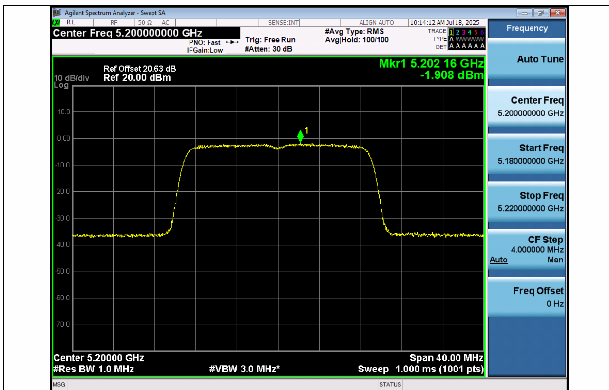
11N20MIMO-Ant1-5200-PASS
