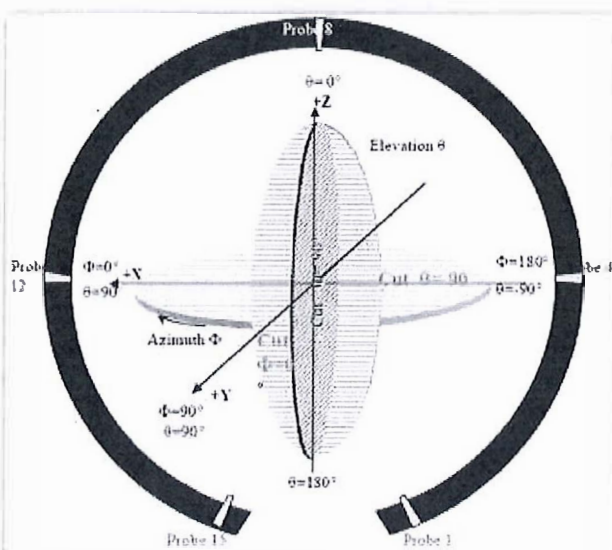
图 1 3D 微波暗室测试坐标系 (back view)
