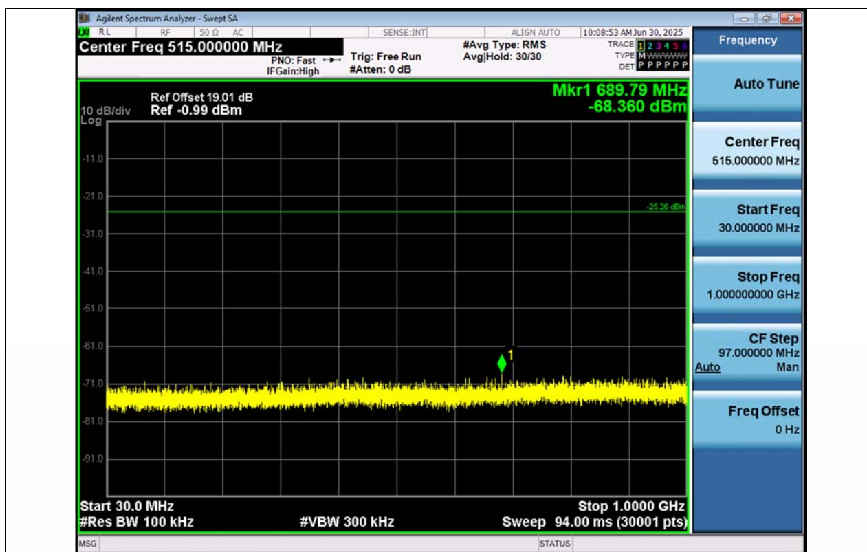
11G-Ant1-2412-30~1000-PASS
