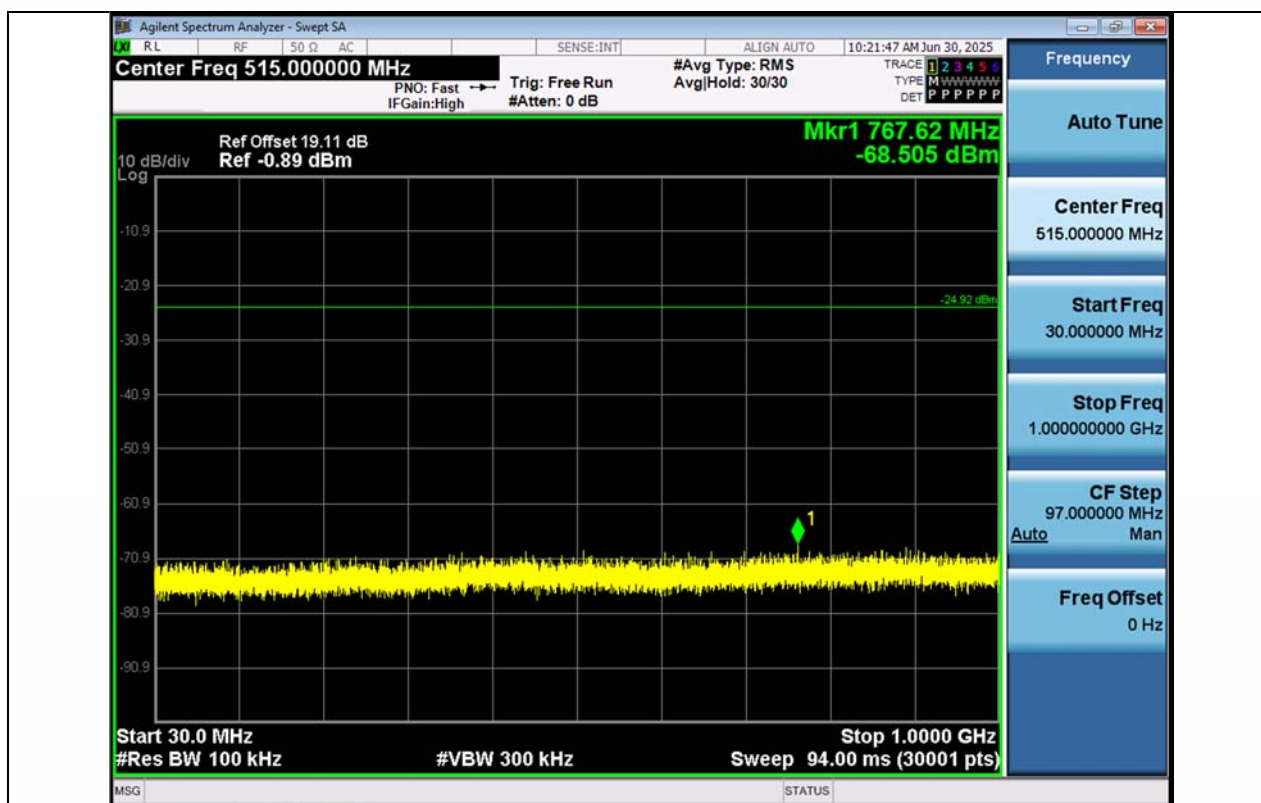
11G-Ant1-2437-30~1000-PASS
