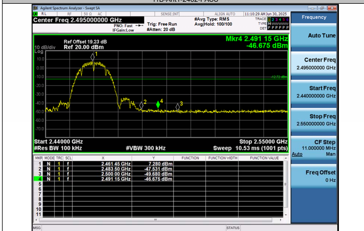
11B-Ant2-2462-PASS
