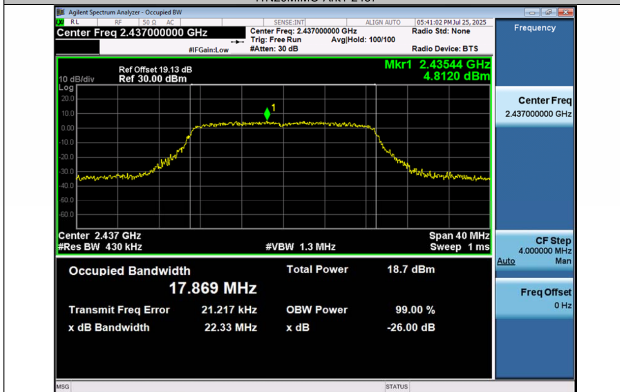
11N20MIMO-Ant2-2437
