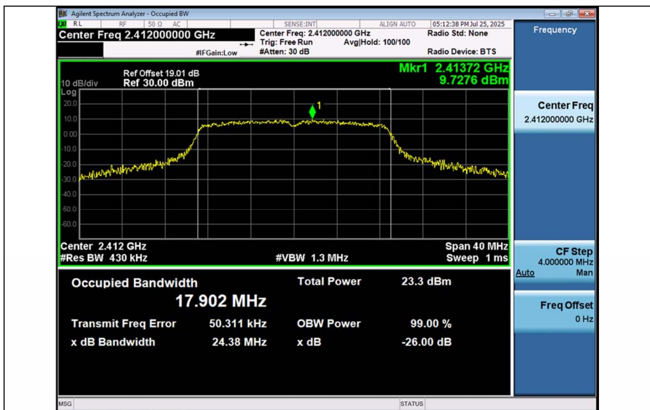
11N20MIMO-Ant1-2412
