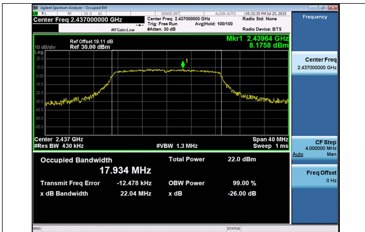
11N20MIMO-Ant1-2437
