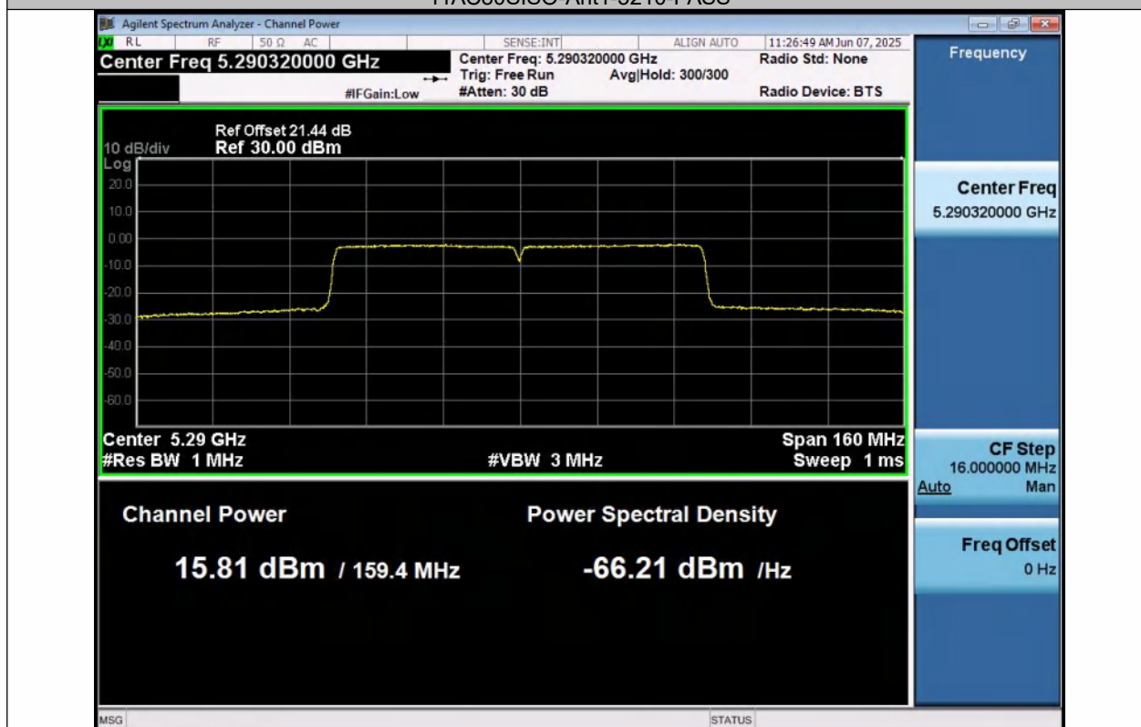
11AC80SISO-Ant1-5290-PASS
