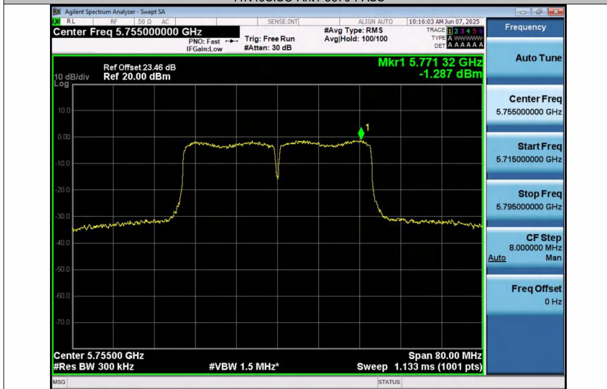
11N40SISO-Ant1-5755-PASS
